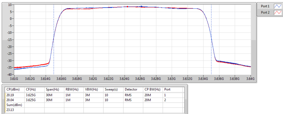
Band 48_LTE_20MHz_Nss1,QPSK_2TX 3625MHz_QPSK_RB 100,#RB 0
