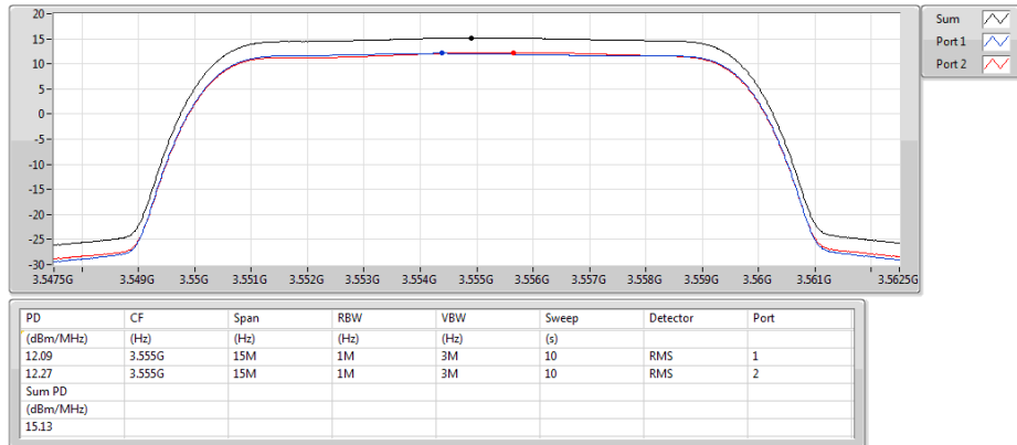
Band 48_LTE_10MHz_Nss1,QPSK_2TX 3555MHz_QPSK_RB 50,#RB 0
