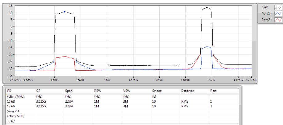
Band 48_LTE_20MHz+10MHz_Nss1,64QAM_2TX P#3560MHz,#3695MHz_64QAM_RB 100,#RB 0+RB 50,#RB 0
