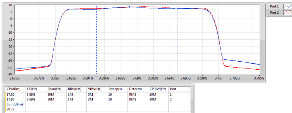
Band 48_LTE_20MHz_Nss1,QPSK_2TX 3690MHz_QPSK_RB 100,#RB 0
