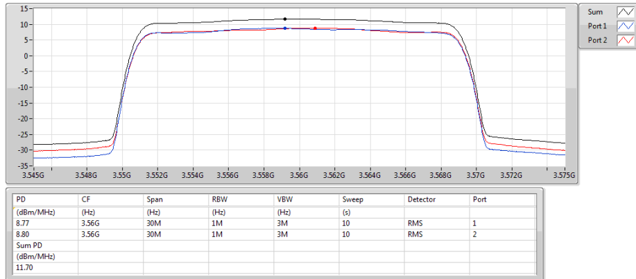
Band 48_LTE_20MHz_Nss1,QPSK_2TX 3560MHz_QPSK_RB 100,#RB 0
