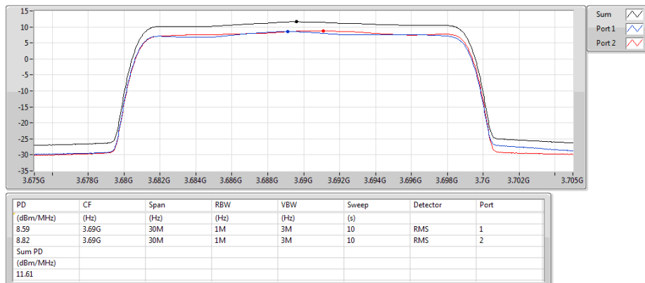
Band 48_LTE_20MHz_Nss1,QPSK_2TX 3690MHz_QPSK_RB 100,#RB 0
