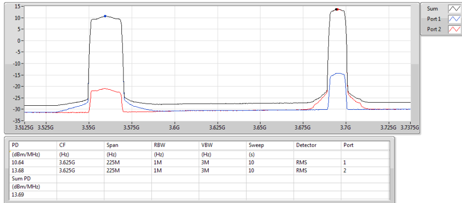
Band 48_LTE_20MHz+10MHz_Nss1,QPSK_2TX P#3560MHz,#3695MHz_QPSK_RB 100,#RB 0+RB 50,#RB 0
