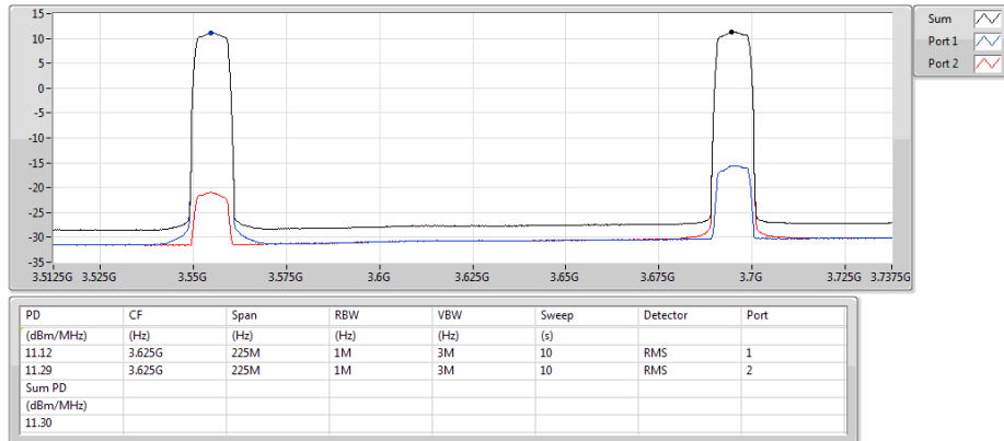
Band 48_LTE_10MHz+10MHz_Nss1,QPSK_2TX P#3555MHz,#3695MHz_QPSK_RB 50,#RB 0+RB 50,#RB 0
