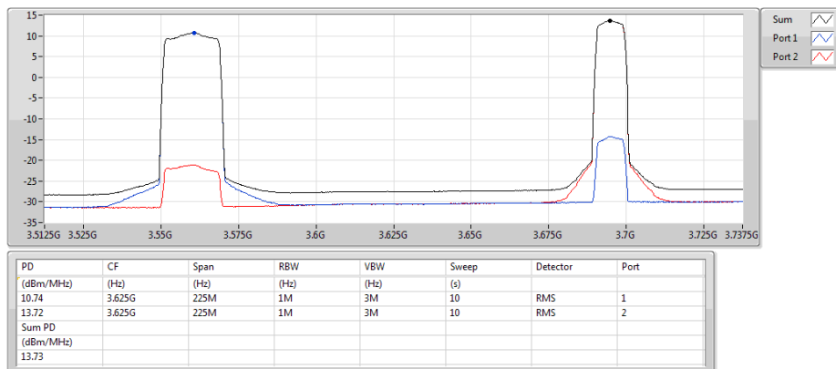
Band 48_LTE_20MHz+10MHz_Nss1,16QAM_2TX P#3560MHz,#3695MHz_16QAM_RB 100,#RB 0+RB 50,#RB 0
