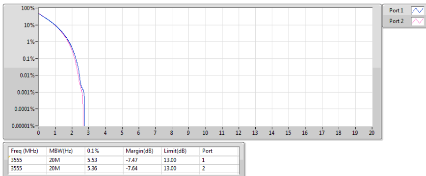
Band 48_LTE_10MHz_Nss1,QPSK_2TX 3555MHz_QPSK_RB 50,#RB 0
