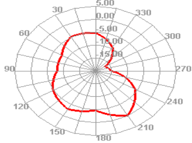
1880.000MHz E1
