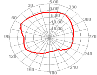
2310.000MHz E2
