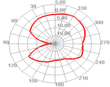
2310.000MHz E1
