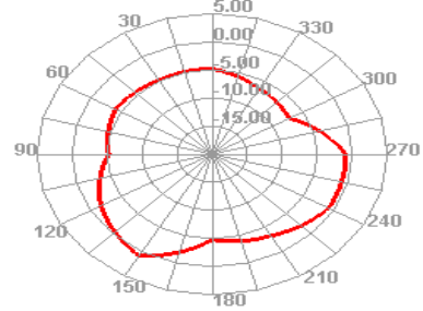
1880.000MHz E2
