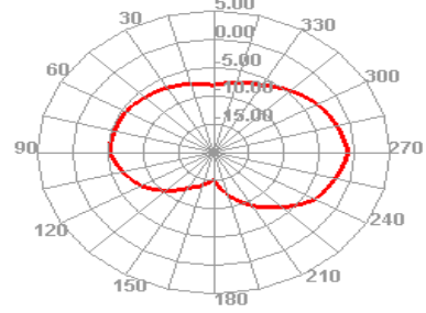
1880.000MHz H
