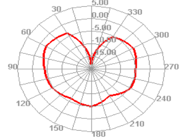
2310.000MHz H
