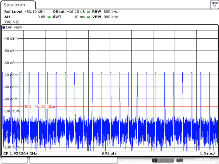
35 µs Pulses
