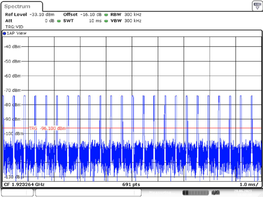
50 µs Pulses
