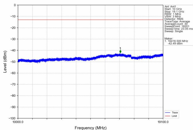
Band2_3MHz_QPSK_HCH_1908.5MHz_RB_1_14_NTNV
