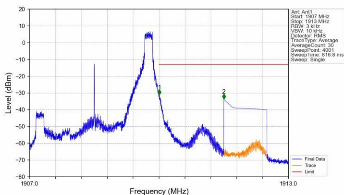
Band2_3MHz_QPSK_HCH_1908.5MHz_RB_1_14_NTNV
