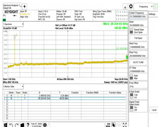
11G_Ant1_2462_1000~26500
