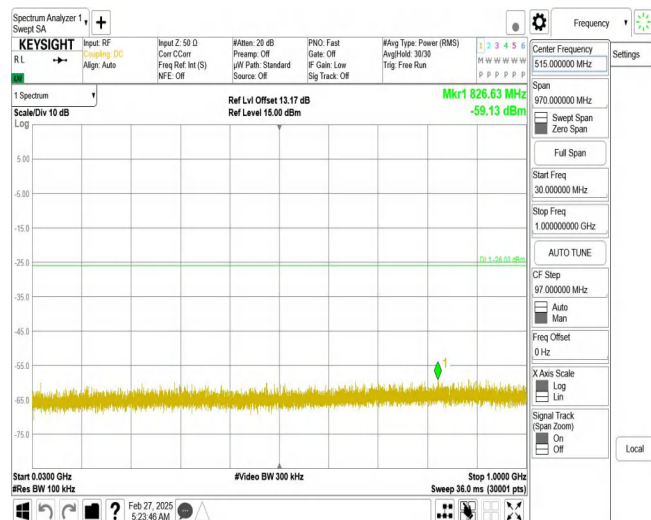
11G_Ant1_2462_30~1000
