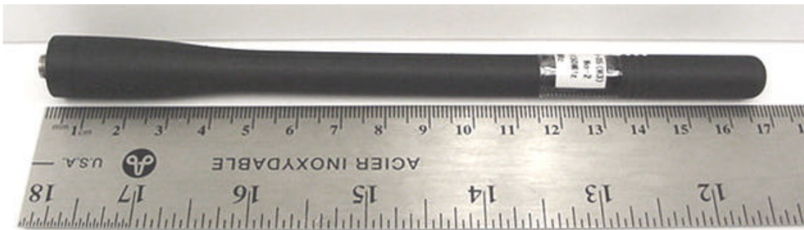
Antenna P/N: KRA-26(M2)
