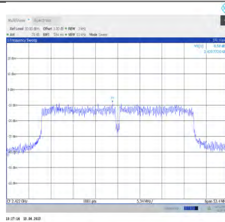
11n40ISO-Ant0-2422
