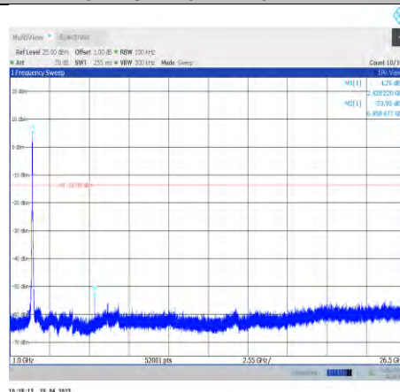
11n40SISO-Ant0-2422-1000~26500
