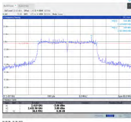
11n40SISO-Ant0-2437
