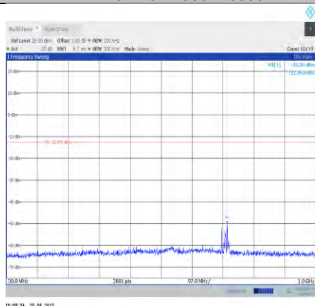
11g-Ant0-2412-30~1000
