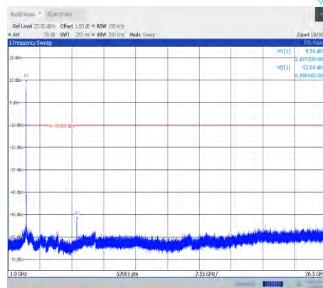
11b-Ant0-2437-1000~26500
