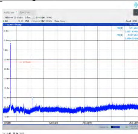
11g-Ant0-2437-1000~26500
