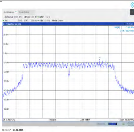
11n20ISO-Ant0-2462
