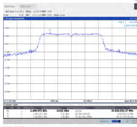
11n40SISO-Ant0-2422
