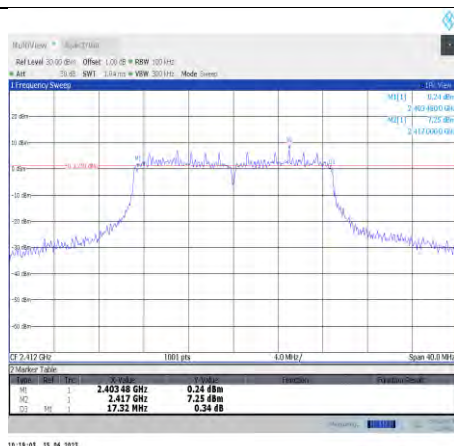
11n20SISO-Ant0-2412
