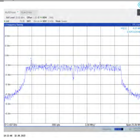
11n20ISO-Ant0-2437
