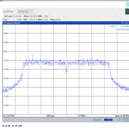
11n20ISO-Ant0-2412
