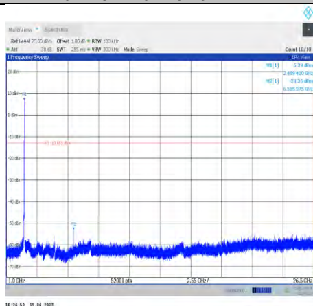
11n20SISO-Ant0-2462-1000~26500
