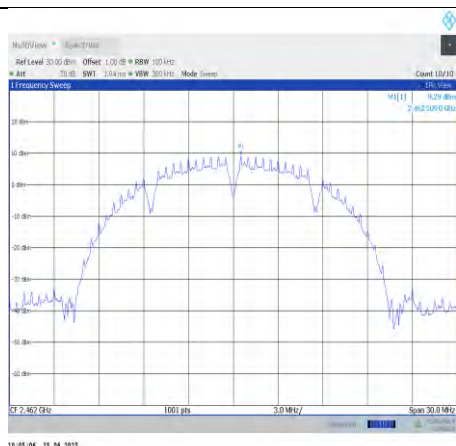
11b-Ant0-2462-0~Reference
