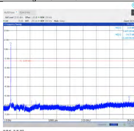
11g-Ant0-2412-1000~26500
