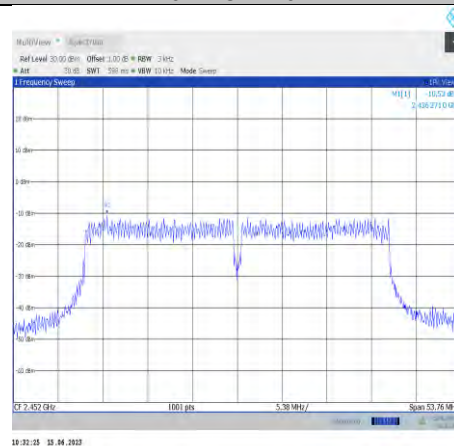
11n40ISO-Ant0-2452
