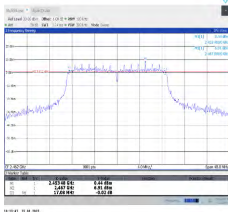
11n20SISO-Ant0-2462
