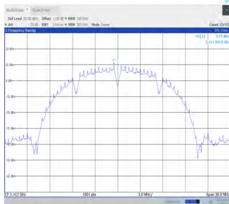
11b-Ant0-2412-0~Reference
