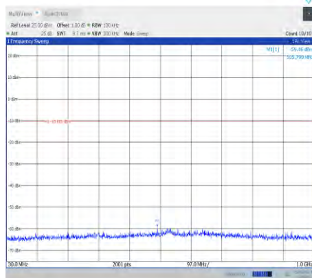
11b-Ant0-2437-30~1000
