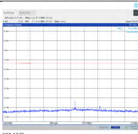
11n40SISO-Ant0-2422-30~1000
