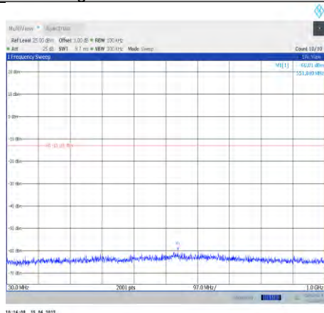
11g-Ant0-2462-30~1000
