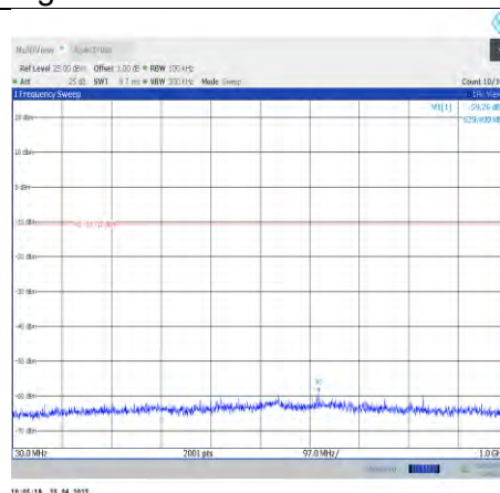
11b-Ant0-2462-30~1000
