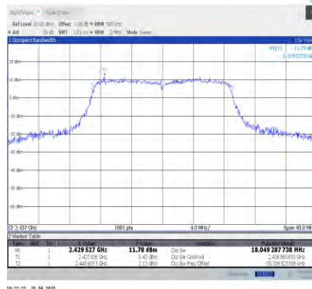
11n20SISO-Ant0-2437
