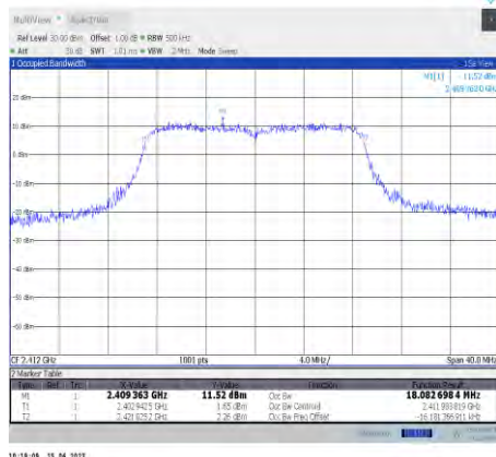
11n20SISO-Ant0-2412
