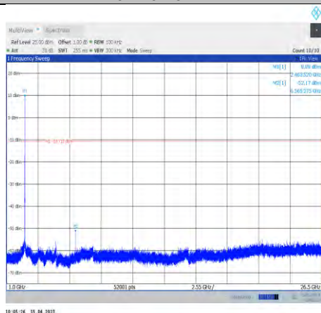
11b-Ant0-2462-1000~26500
