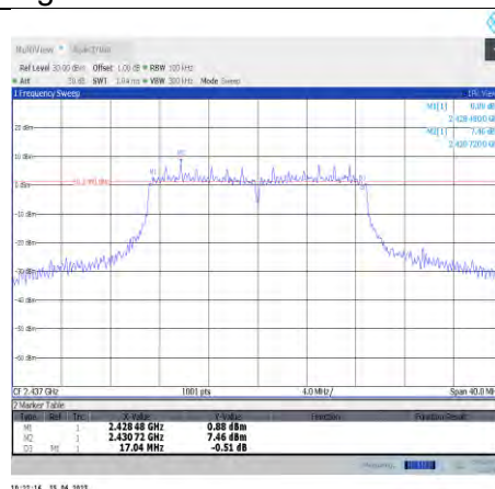
11n20SISO-Ant0-2437
