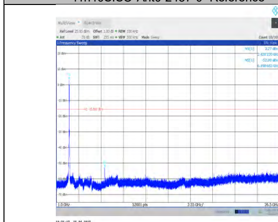
11n40SISO-Ant0-2437-1000~26500
