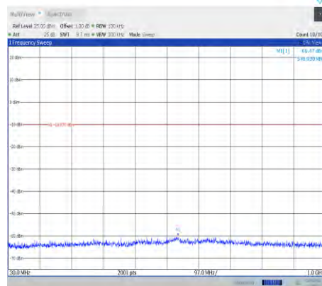
11b-Ant0-2412-30~1000
