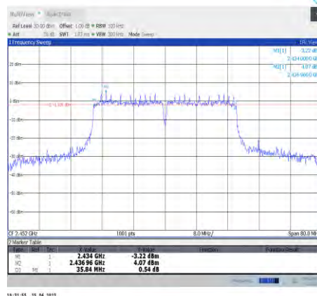
11n40SISO-Ant0-2452
