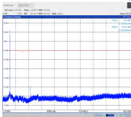
11b-Ant0-2412-1000~26500
