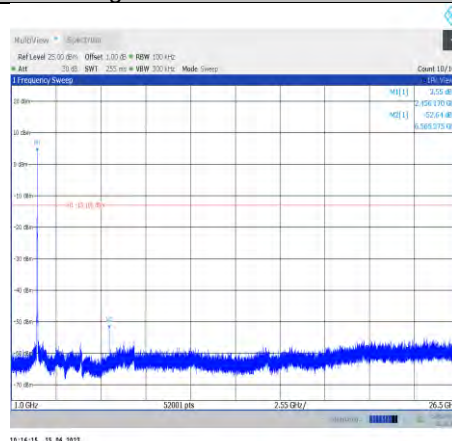
11g-Ant0-2462-1000~26500
