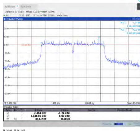
11n40SISO-Ant0-2422
