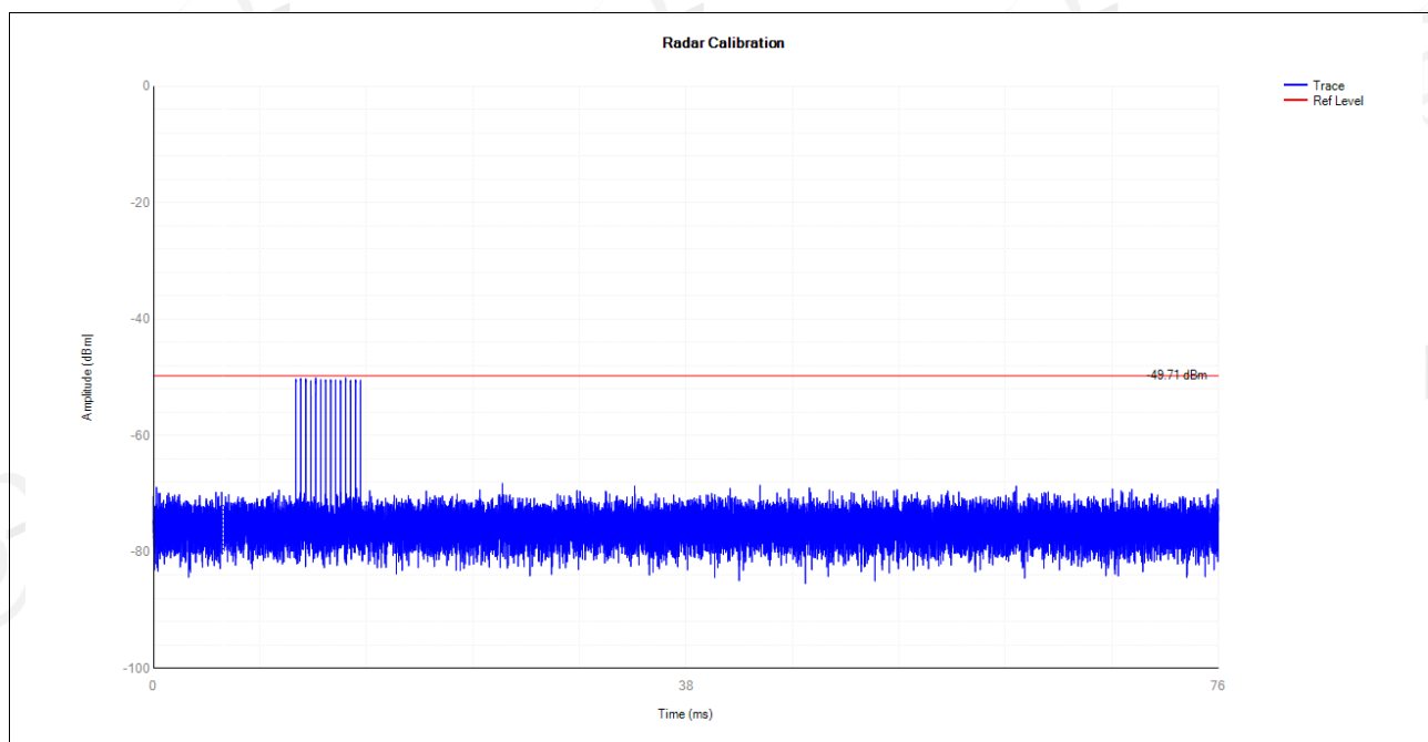
5700MHz DFS_FCC_T5000
