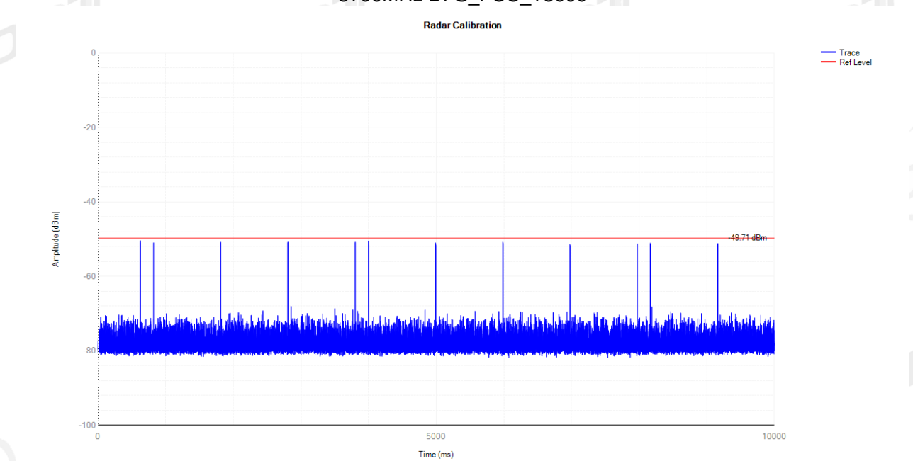
5700MHz DFS_FCC_T6000
