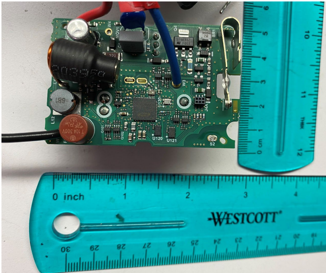
Bottom PCB
