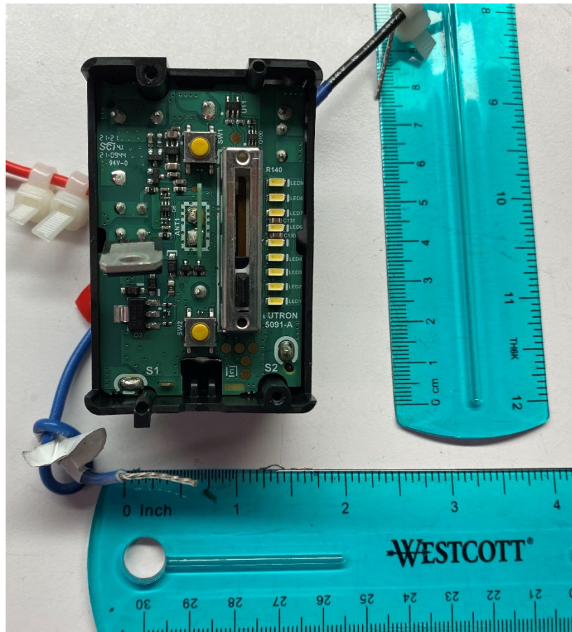
Top PCB
