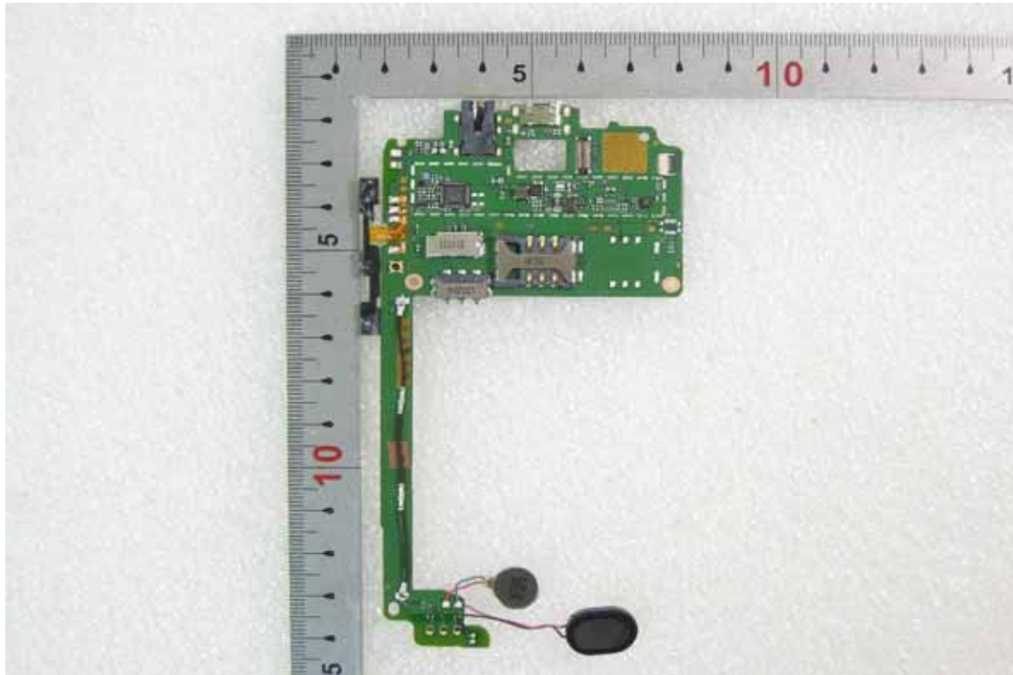
WWAN Antenna
