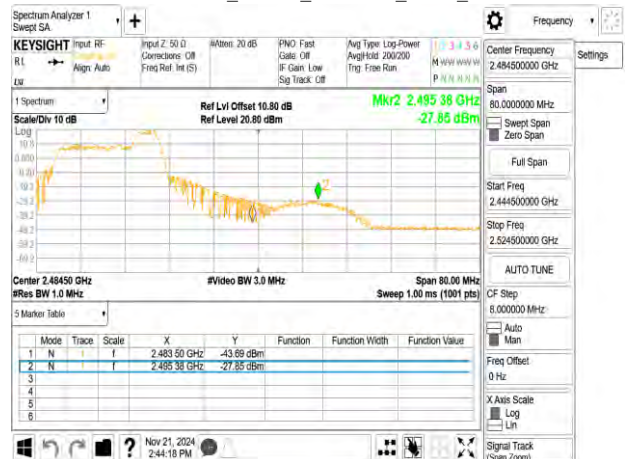
802.11ax_20MHz_2462MHz
