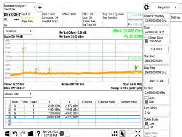
802.11ax_40MHz_Chain0_2452MHz_RU484
