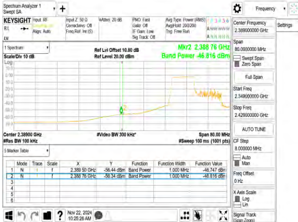
802.11ax_20MHz_2417MHz_RU242
