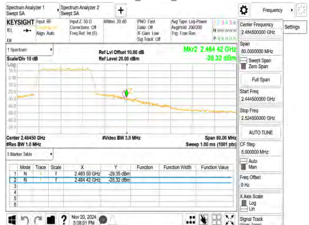
802.11ax_20MHz_2462MHz
