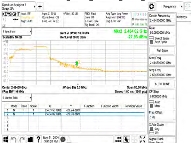
802.11ax_20MHz_2457MHz_RU242RU242
