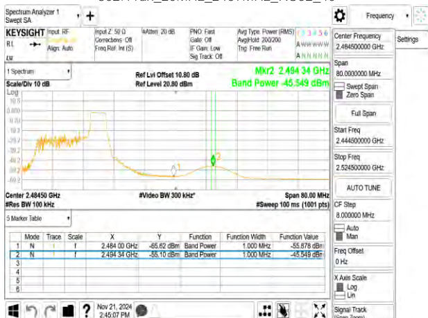
802.11ax_20MHz_2457MHz_RU52_40
