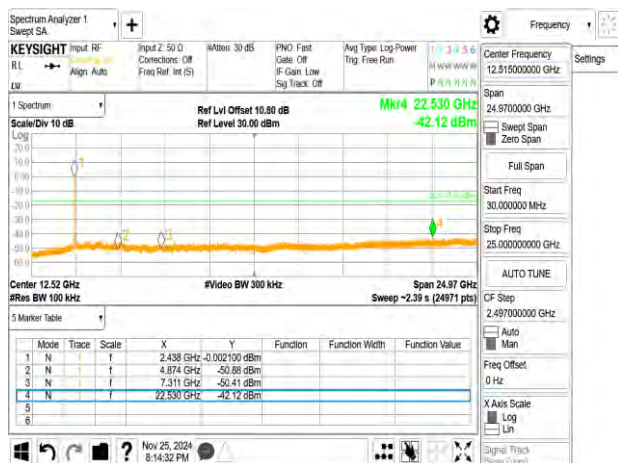
802.11ax_40MHz_Chain0_2437MHz_RU484
