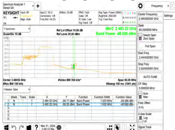
802.11ax_20MHz_2462MHz_RU242
