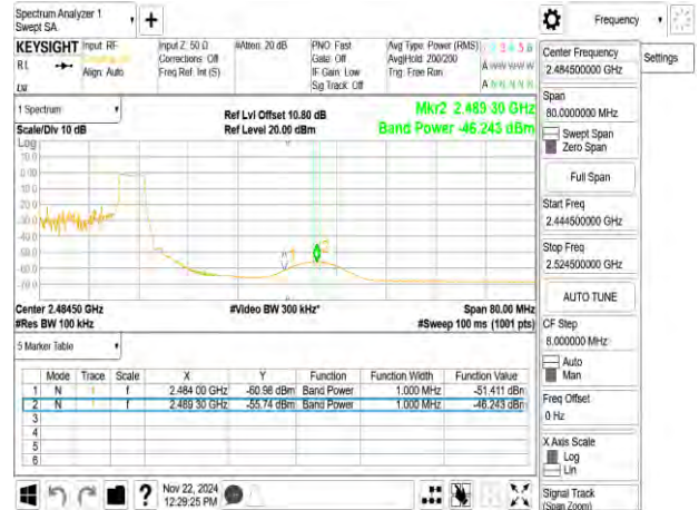
802.11ax_20MHz_2457MHz
