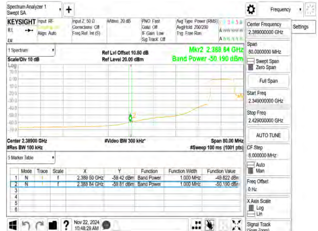
802.11ax_20MHz_2427MHz_RU242
