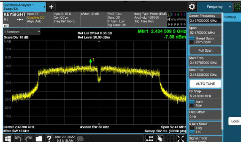
11N40MIMO Ant2 2437
