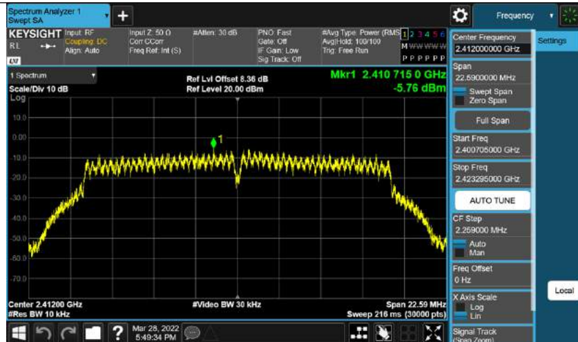
11G_Ant2_2412
