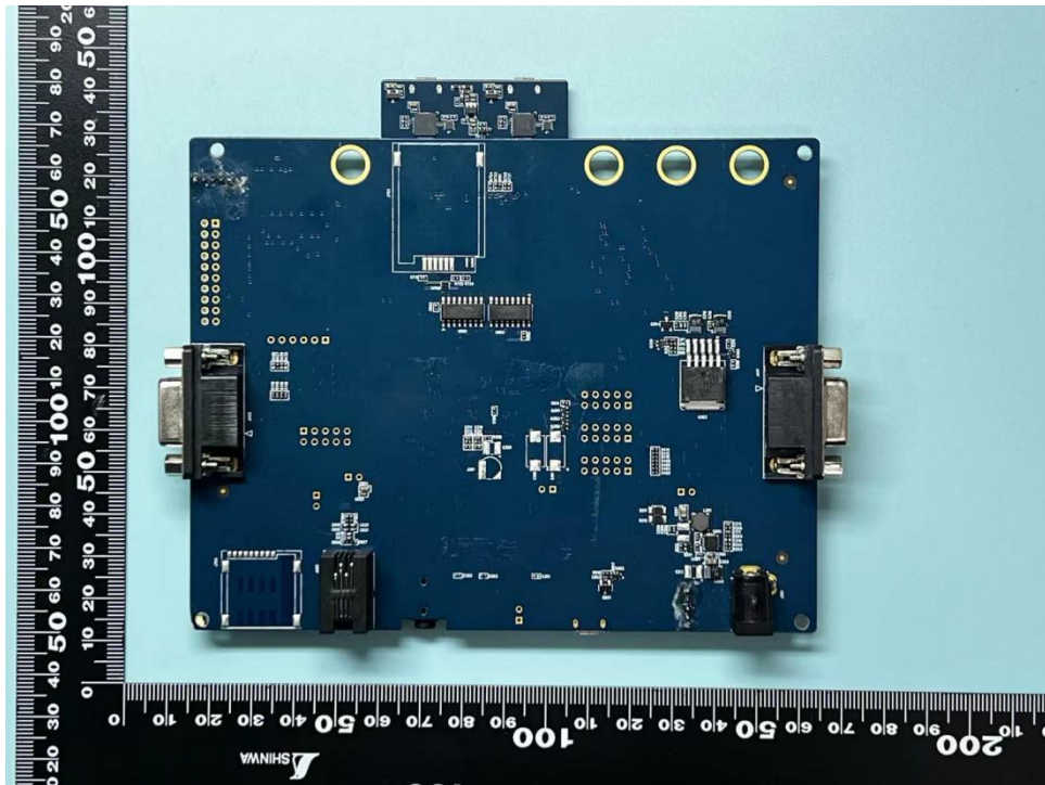
EG916Q-GL + EVB_Bottom
