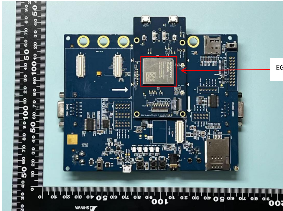
EG916Q-GL + EVB_Top
