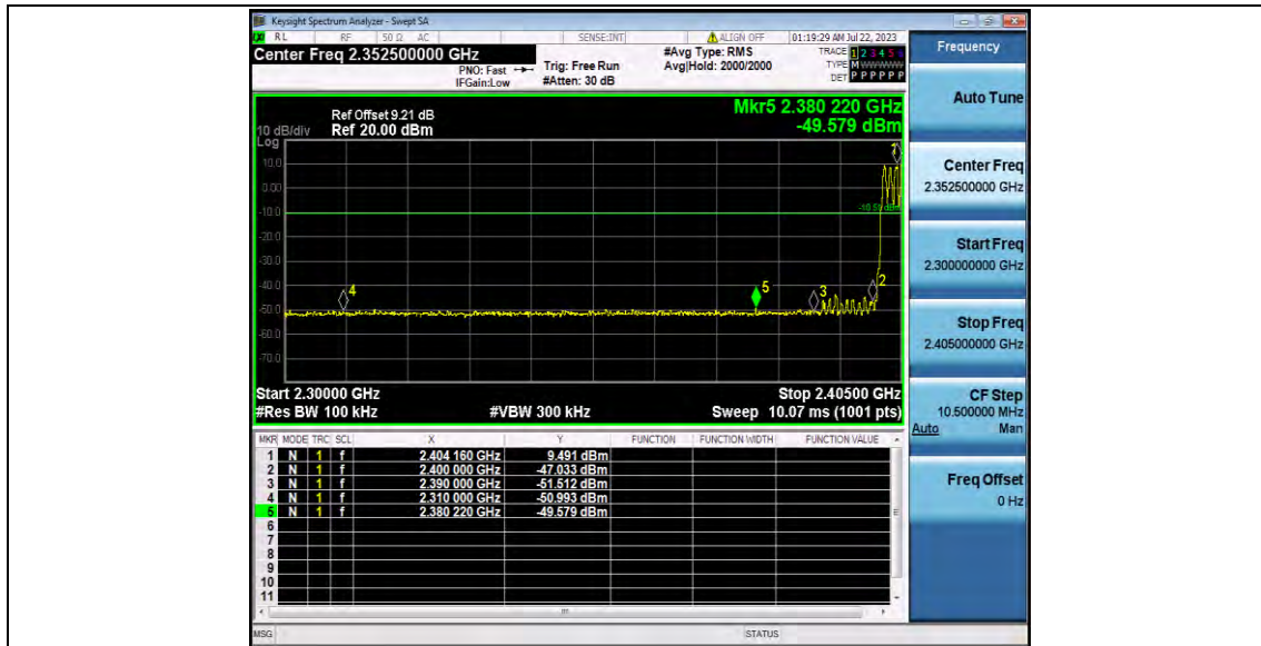
DH1_Ant0_Low_Hop_2402
