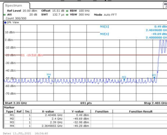
DH1 Ant0 Low Hop 2402
