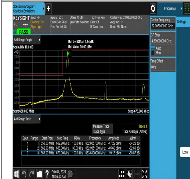
Band71_10MHz_QPSK_133172_1RB#0
