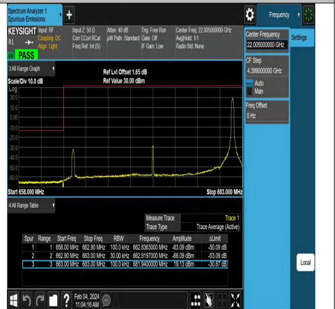
Band71_20MHz_QPSK_133222_1RB#99
