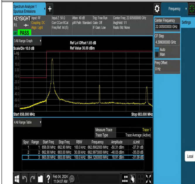
Band71_20MHz_QPSK_133222_1RB#0
