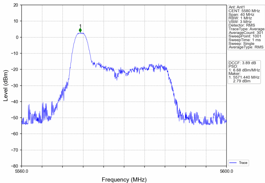
802.11ax(HEW20)_MCH_5580MHz_RU26_Left_Ant1_NTNV
