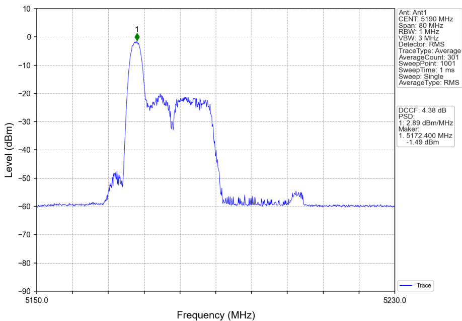
802.11ax(HEW40)_LCH_5190MHz_RU26_Left_Ant1_NTNV
