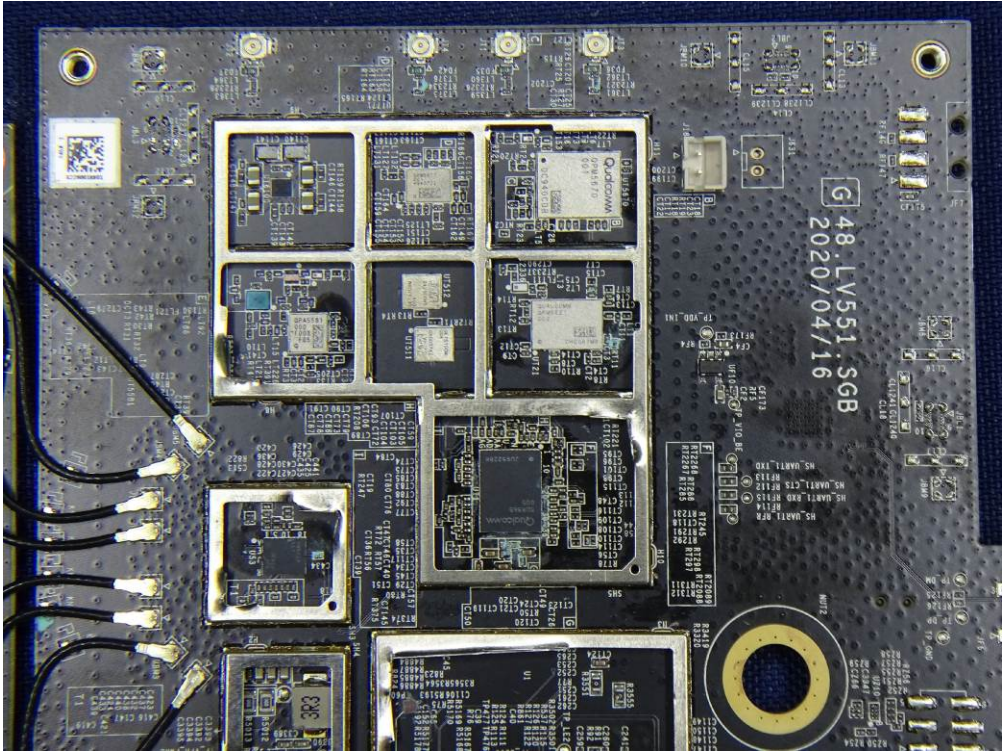
(95) EUT Photo
