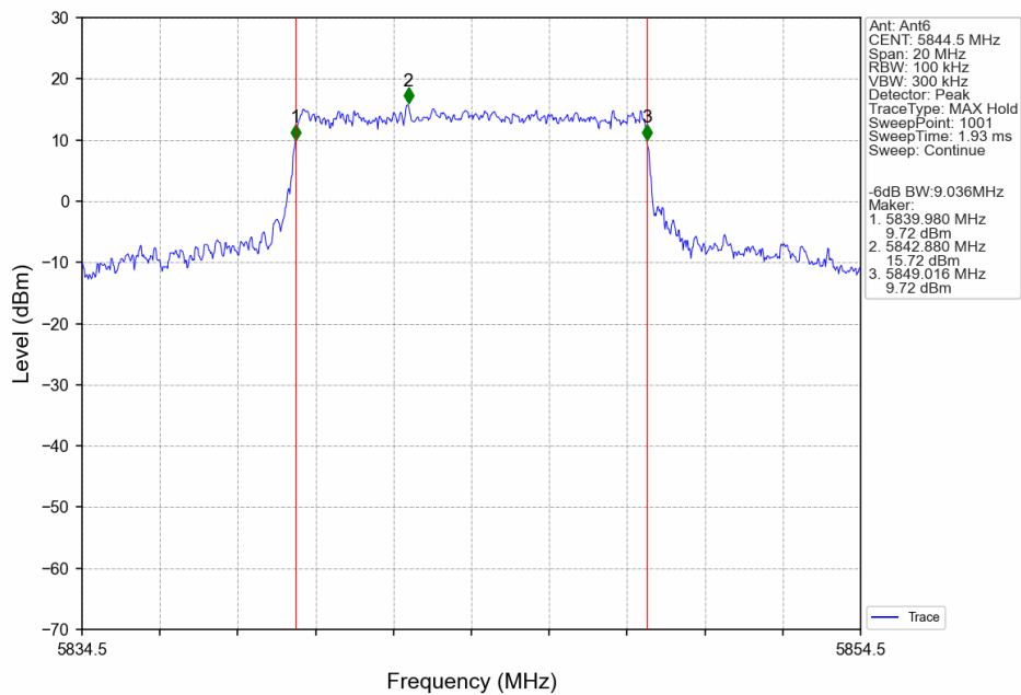
10M_HCH_5844.5MHz_Ant6_NTNV
