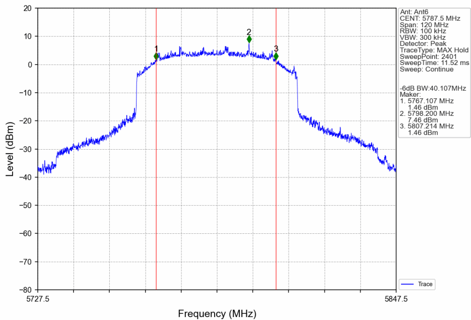
60M_MCH_5787.5MHz_Ant6_NTNV
