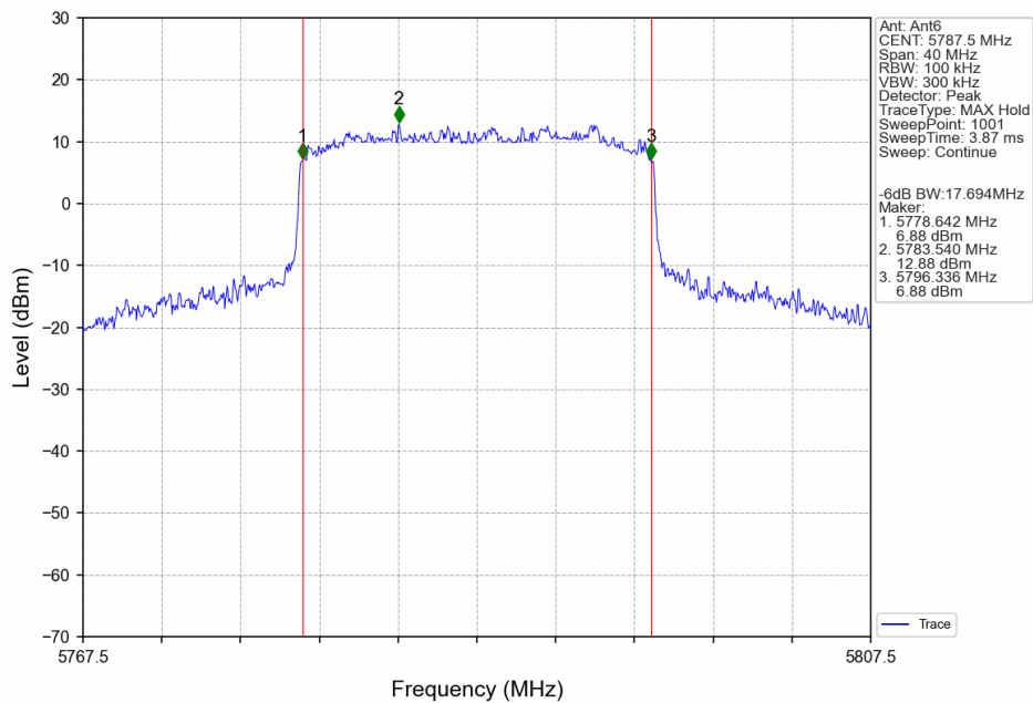
20M_MCH_5787.5MHz_Ant6_NTNV
