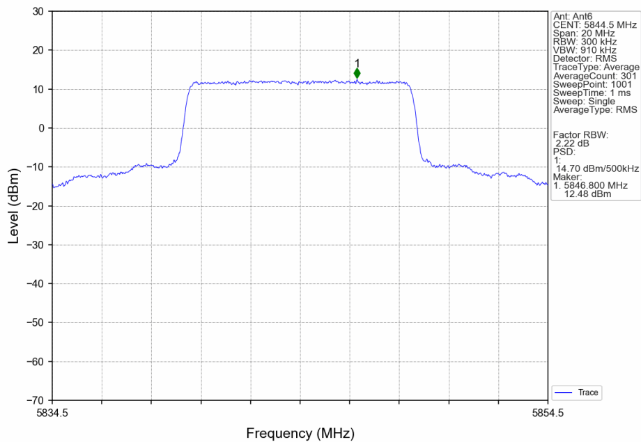
10M_HCH_5844.5MHz_Ant6_NTNV
