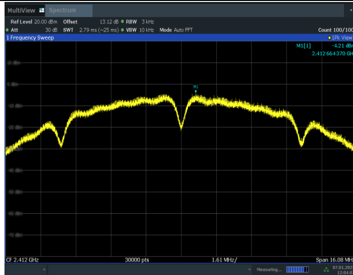
11B_Ant1_2412
