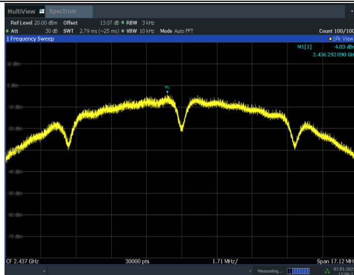
11B_Ant1_2437
