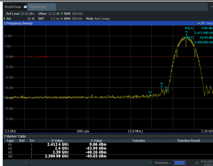
11B_Ant1_Low_2412
