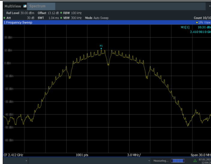
11B_Ant1_2412_0~Reference
