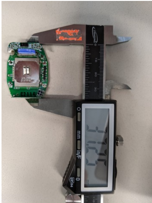
7.6 EUT _ PCB Dimensions
