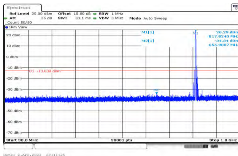
Band26-3MHz-16QAM-26740-1-0-Low-30-1000--34.34-PASS
