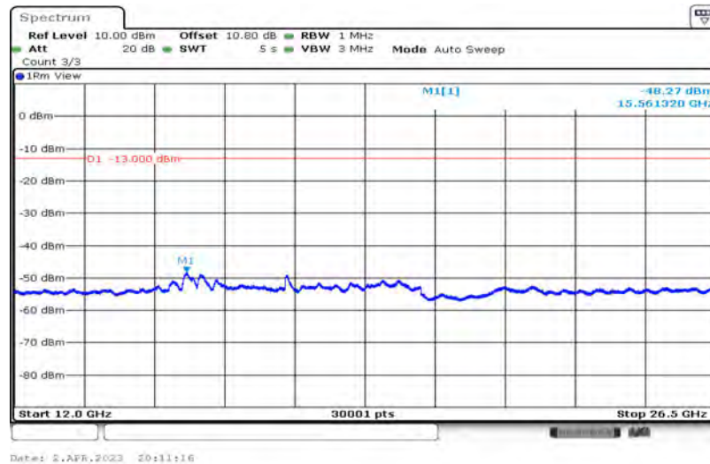
Band26-3MHz-16QAM-26740-1-0-Low-30-1000--34.34-PASS
