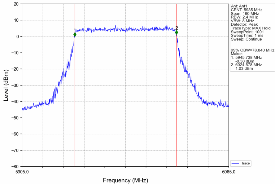
802.11ax(HEW80)_LCH_5985MHz_RU996_Left_Ant1_NTNV
