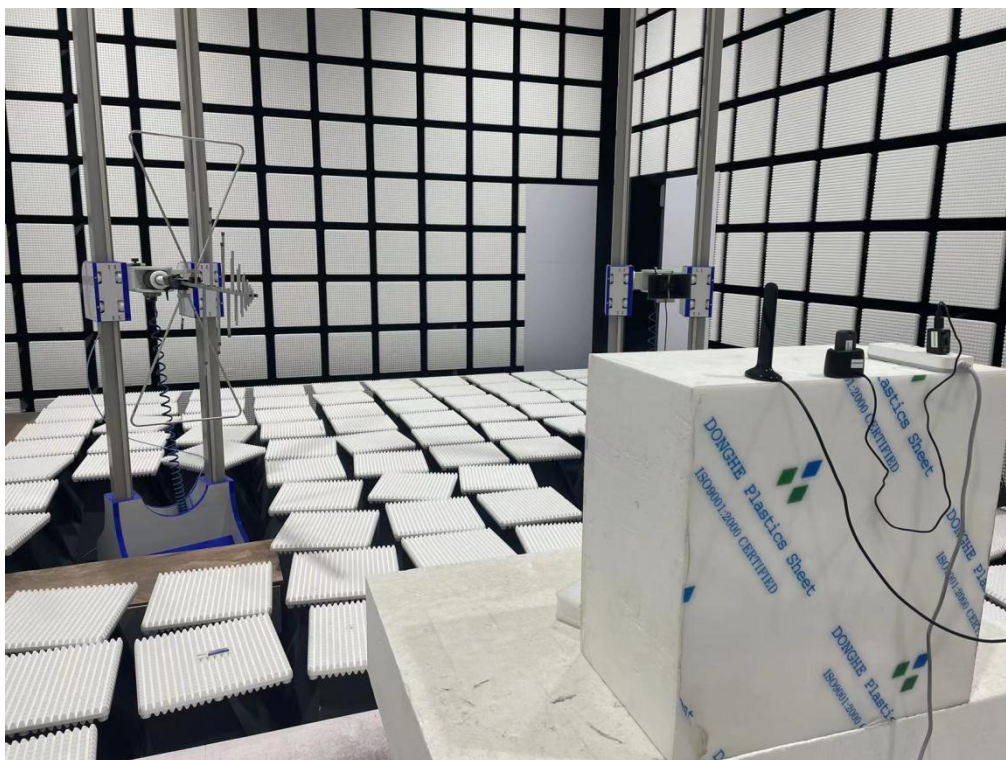
Pic5.RSE(1GHz-18GHz)
