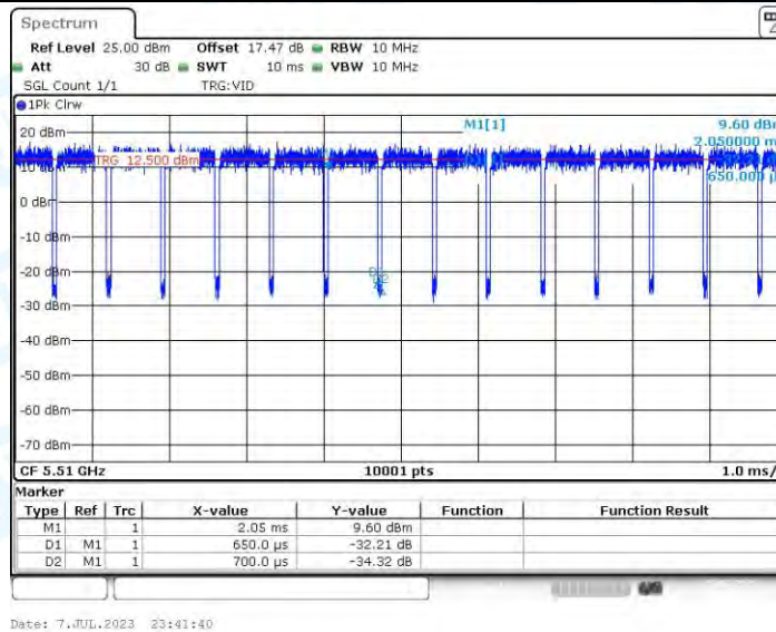
11N40-CDD_Ant3_5510
