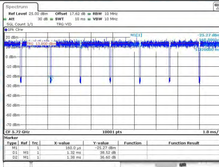
11AC20-CDD_Ant2_5720
