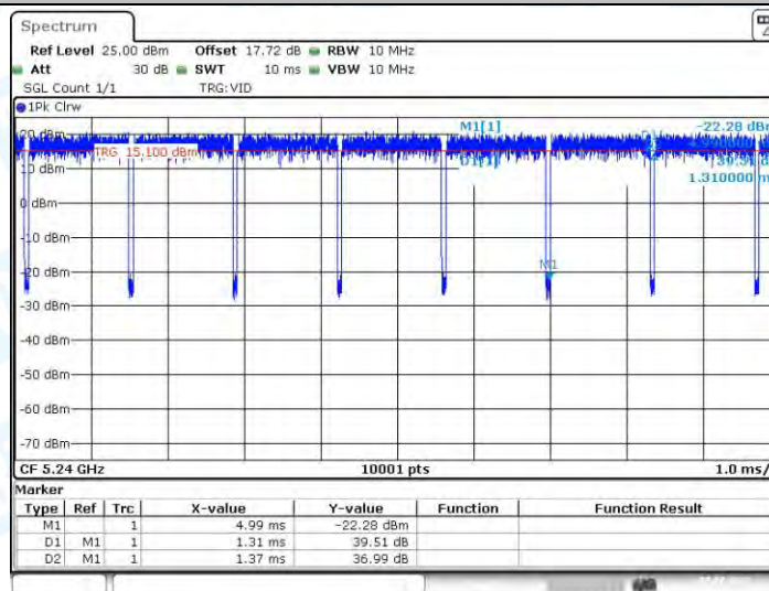
11N20-CDD_Ant3_5240
