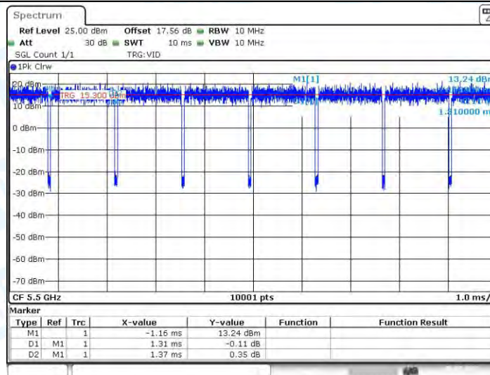
11AC20-CDD_Ant2_5500
