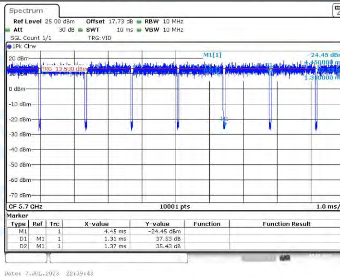
11N20-CDD_Ant4_5700
