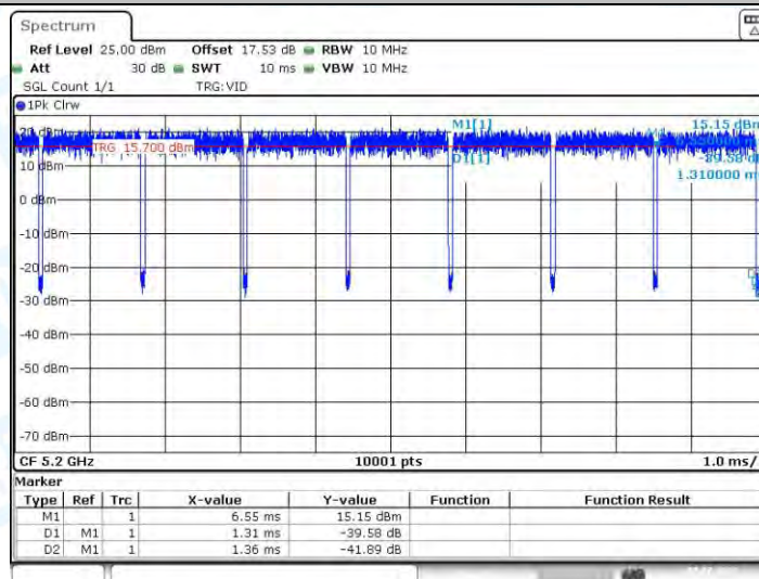
11N20-CDD_Ant4_5200
