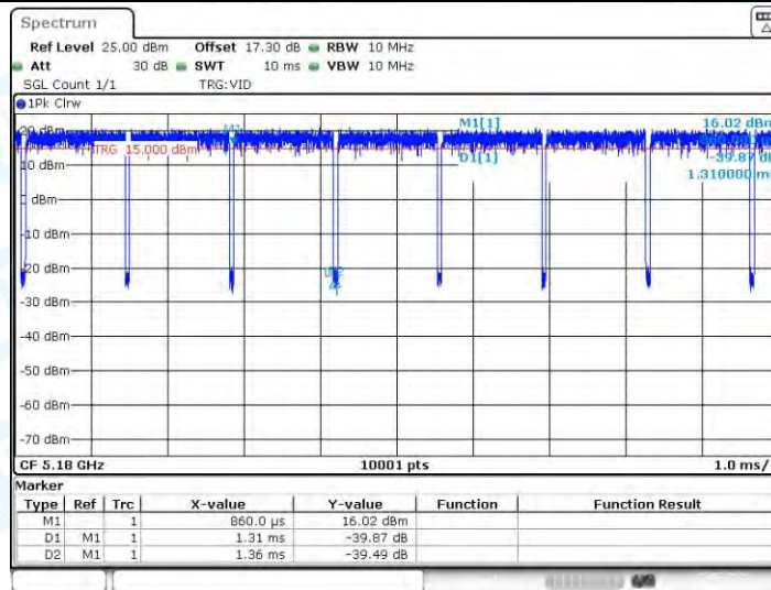
11N20-CDD_Ant1_5180
