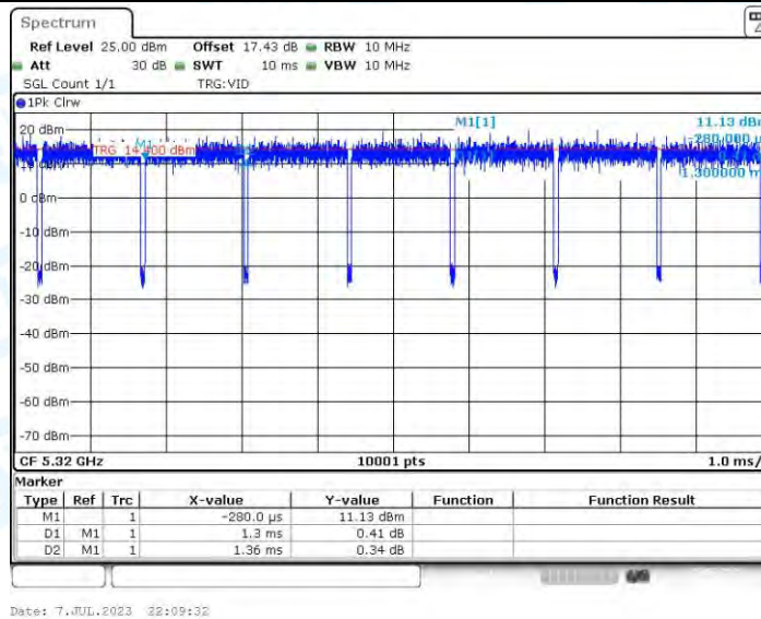
11N20-CDD_Ant3_5320
