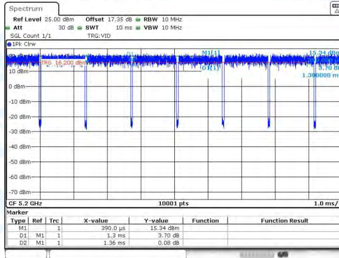
11N20-CDD_Ant3_5200
