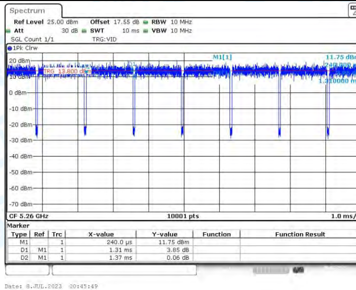
11AC20-CDD_Ant2_5260
