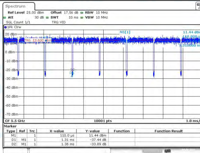
11N20-CDD_Ant2_5500
