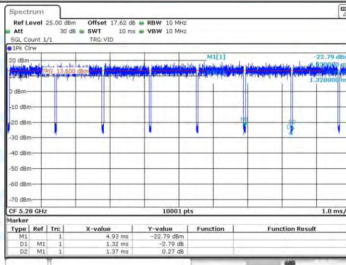
11AC20-CDD_Ant1_5280
