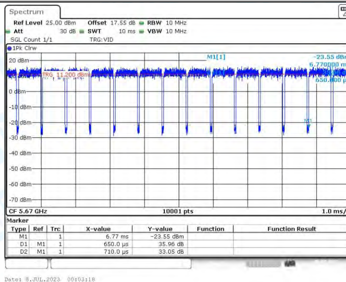
11N40-CDD_Ant2_5670
