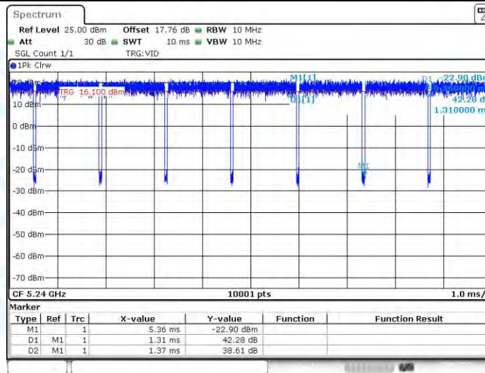
11N20-CDD_Ant2_5240
