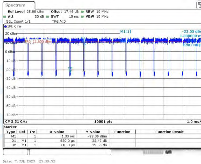
11N40-CDD_Ant2_5510
