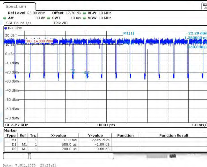
11N40-CDD_Ant3_5270
