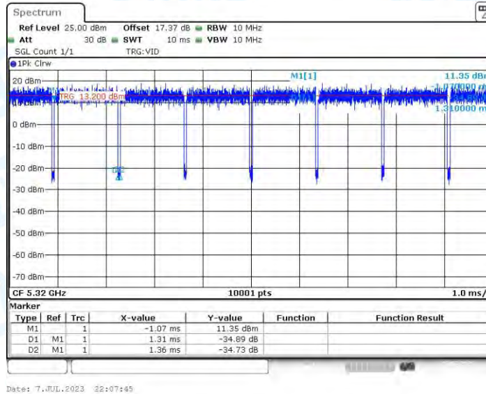
11N20-CDD_Ant2_5320
