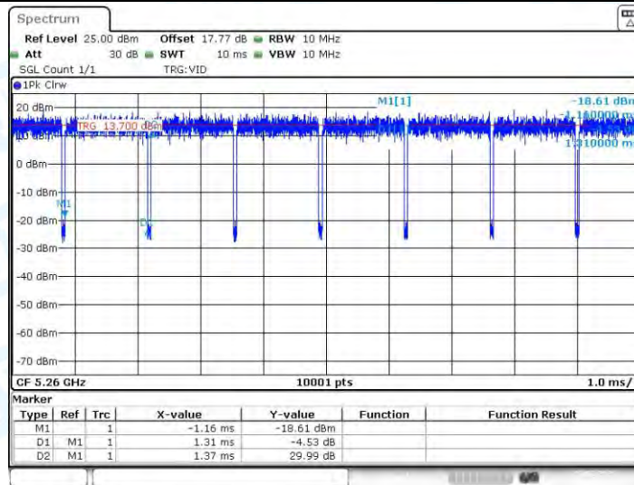
11N20-CDD_Ant4_5260
