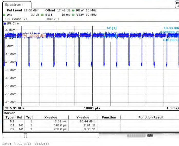
11N40-CDD_Ant3_5310
