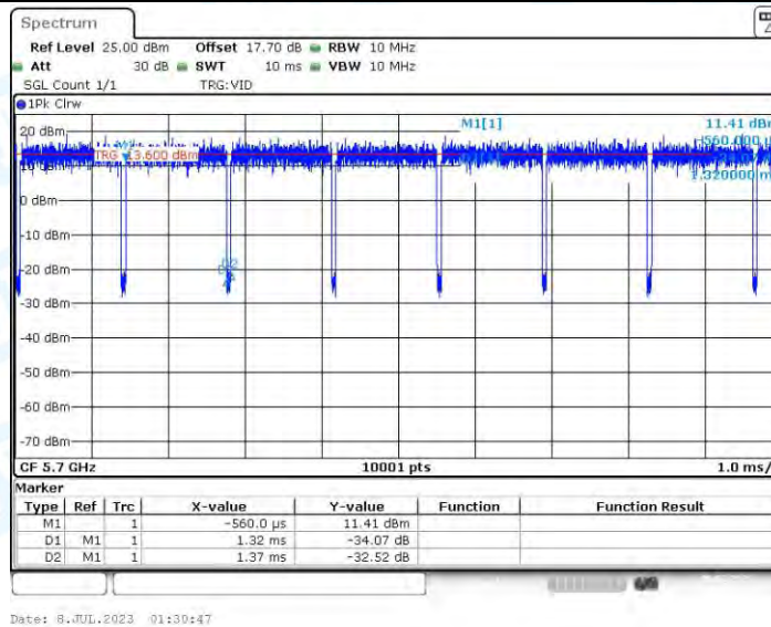
11AC20-CDD_Ant3_5700
