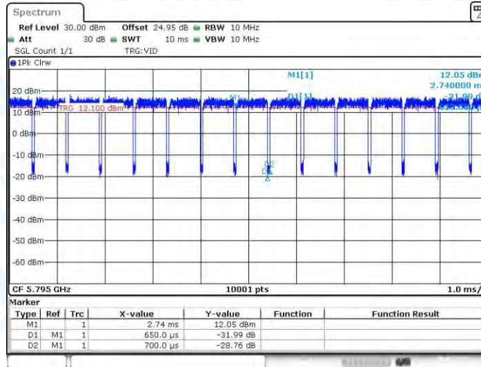
11N40-CDD_Ant2_5795
