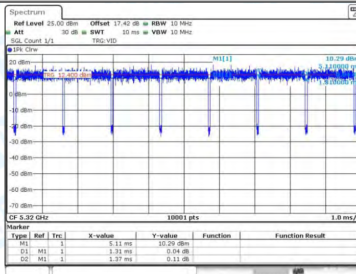
11AC20-CDD_Ant3_5320
