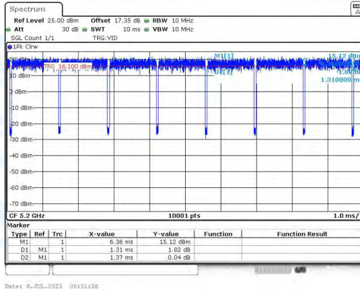
11AC20-CDD_Ant3_5200
