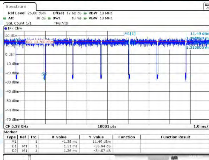
11N20-CDD_Ant1_5280
