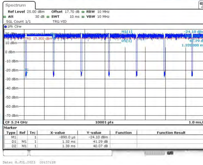
11AC20-CDD_Ant2_5240
