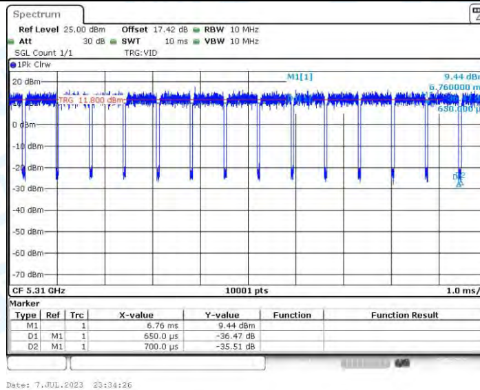
11N40-CDD_Ant4_5310
