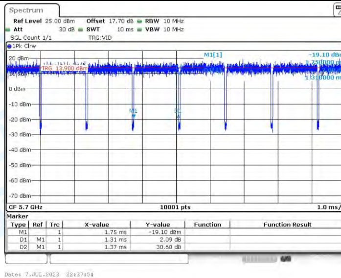
11N20-CDD_Ant3_5700
