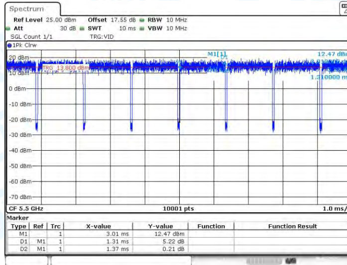
11AC20-CDD_Ant1_5500
