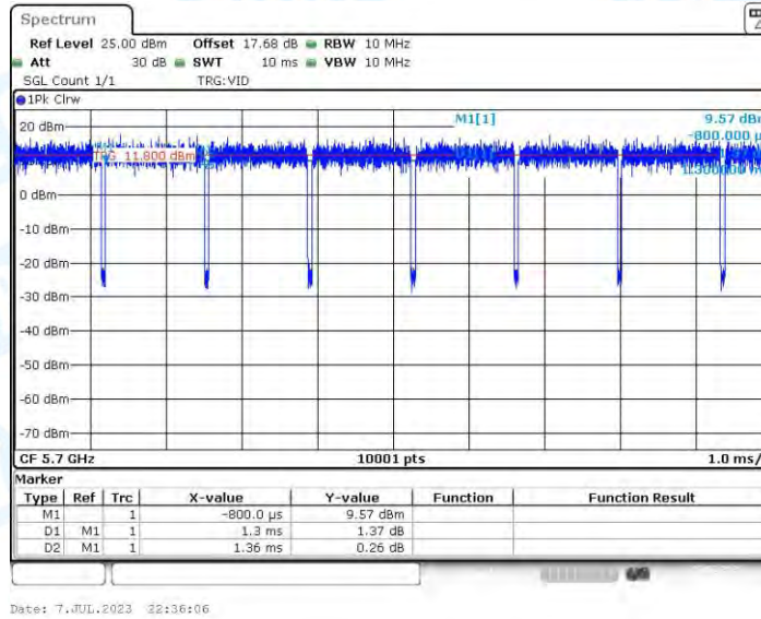
11N20-CDD_Ant2_5700
