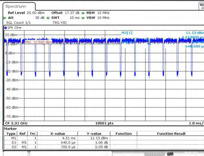
11N40-CDD_Ant1_5310
