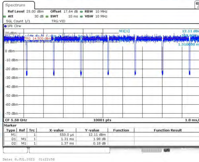
11AC20-CDD_Ant3_5580
