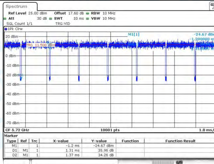
11N20-CDD_Ant1_5720
