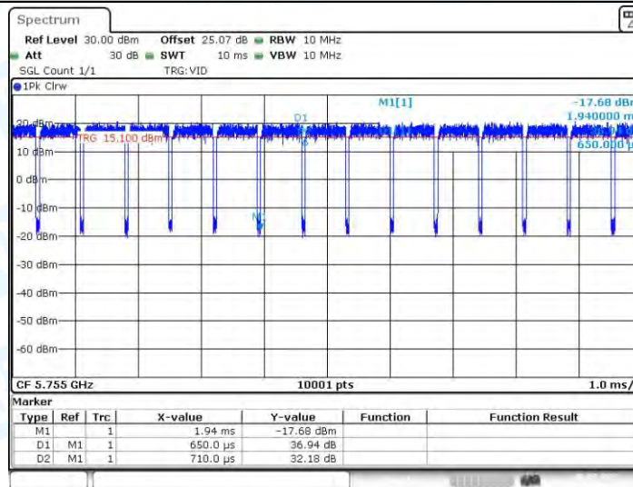
11N40-CDD_Ant4_5755
