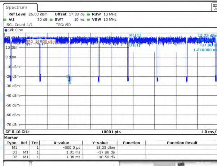
11N20-CDD_Ant2_5180
