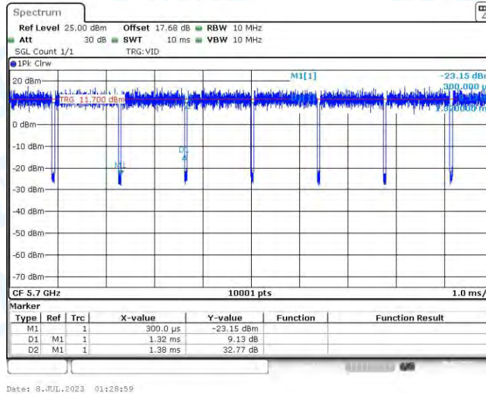
11AC20-CDD_Ant2_5700
