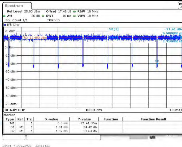
11N20-CDD_Ant4_5320
