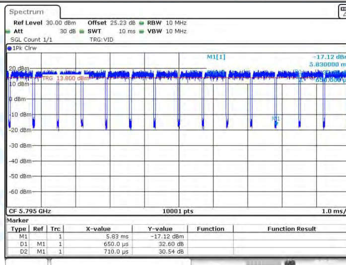
11N40-CDD_Ant3_5795
