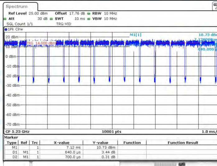
11N40-CDD_Ant2_5230
