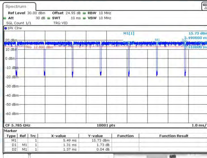
11AC20-CDD_Ant1_5785
