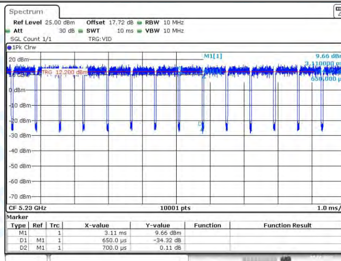
11N40-CDD_Ant3_5230
