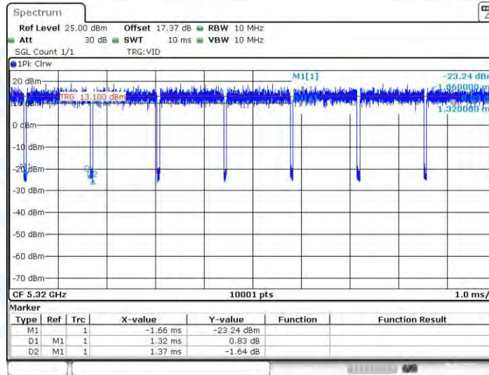
11AC20-CDD_Ant2_5320
