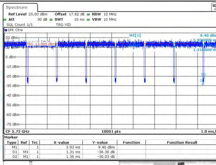
11N20-CDD_Ant2_5720
