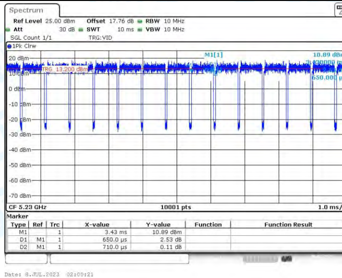
11AC40-CDD_Ant3_5230
