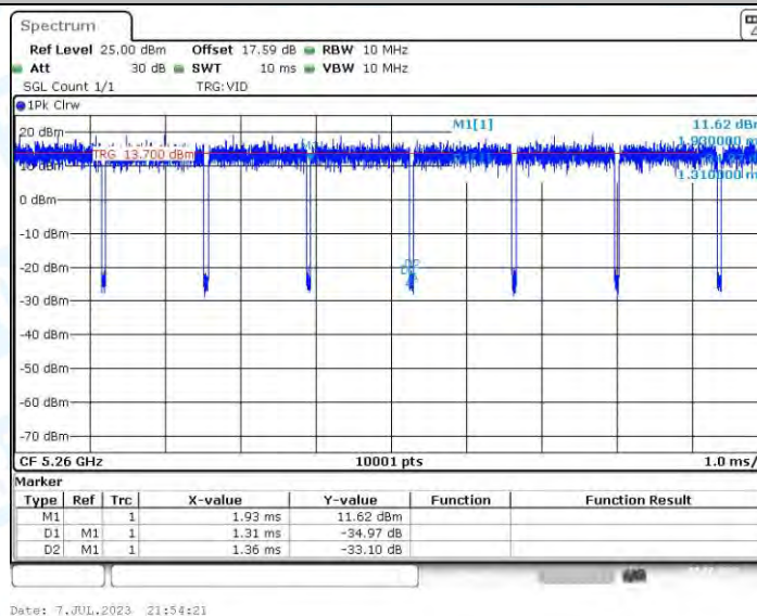
11N20-CDD_Ant3_5260
