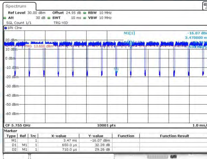
11N40-CDD_Ant3_5755
