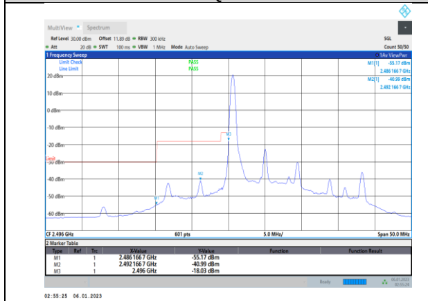
Band41-10MHz-QPSK-39700-50RB#0
