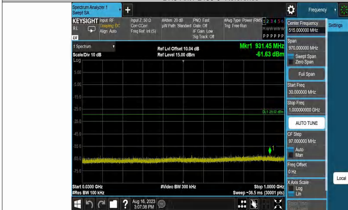
DH5-Ant1-2480-30~1000
