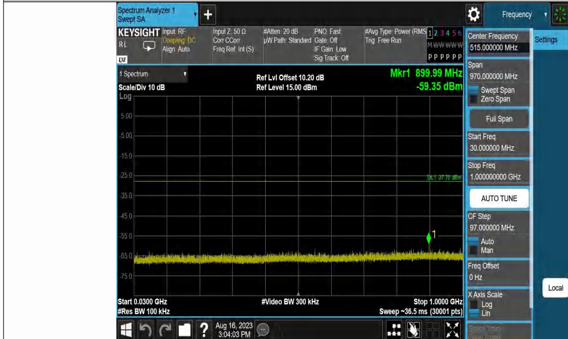
DH5-Ant1-2402-30~1000
