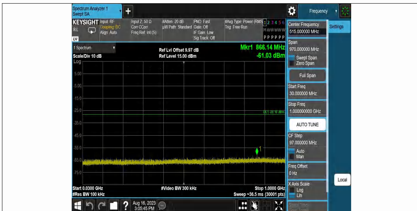
DH5-Ant1-2441-30~1000
