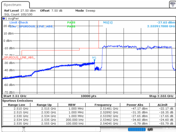
2_20MHz_Low_QPSK_100@0
