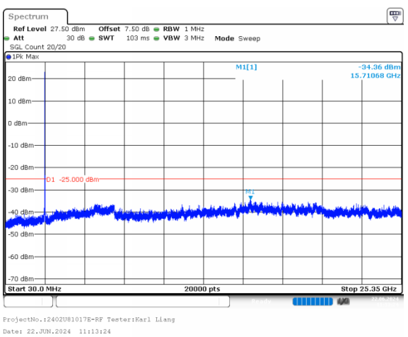
20MHz_Low_QPSK_1@0
