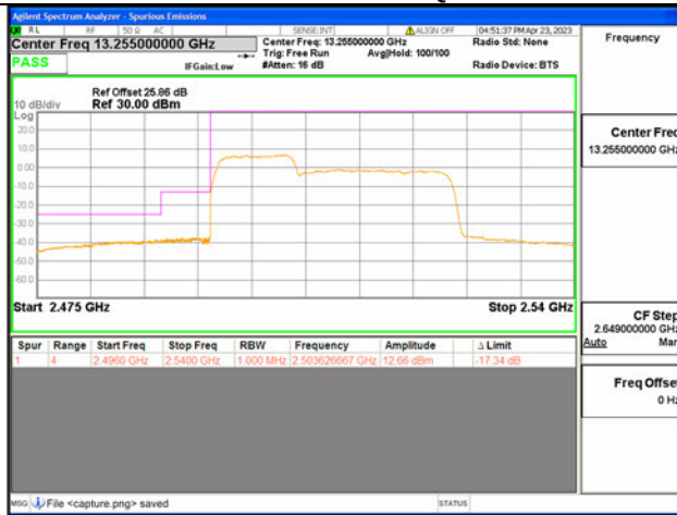
41C / 10+20MHz / Low CH / QPSK / 50#0-100#0
