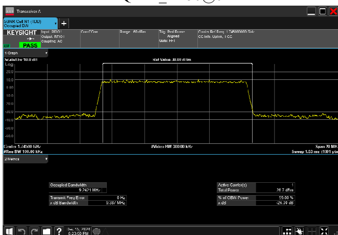
n66_10MHz_15kHz_1745MHz_DFT-s-OFDM QPSK_RB50@0
