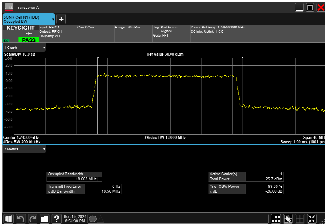
n66_20MHz_15kHz_1745MHz_CP-OFDM QPSK_RB106@0
