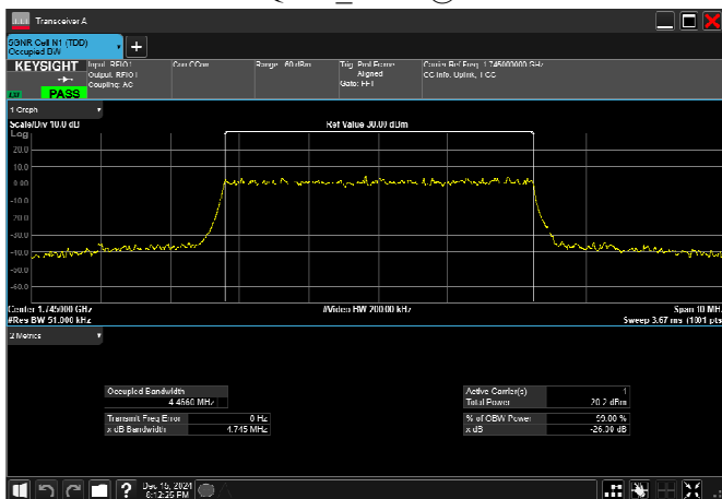
n66_10MHz_15kHz_1745MHz_DFT-s-OFDM QPSK_RB50@0
