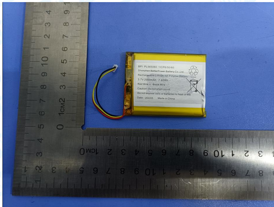
Photo 7 Battery parameters
