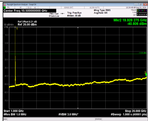
2-2-20MHz-20MHz-QPSK-QPSK-18801-18999-1RB#0-ORB #0-1000~20000MHz-PASS
