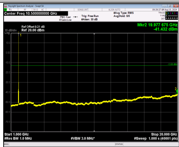
2-2-5MHz-20MHz-QPSK-QPSK-18808-18925-1RB#24-0RB #0-1000~20000MHz-PASS
