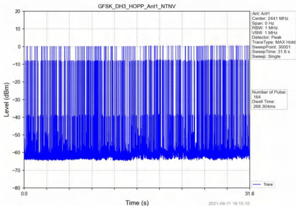
GFSK_DH3_HOPP_Ant1_NTNV
