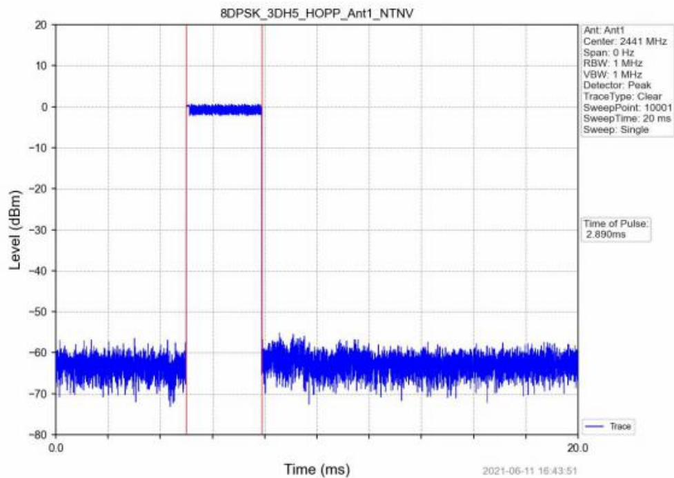
8DPSK_3DH5_HOPP_Ant1_NTNV
