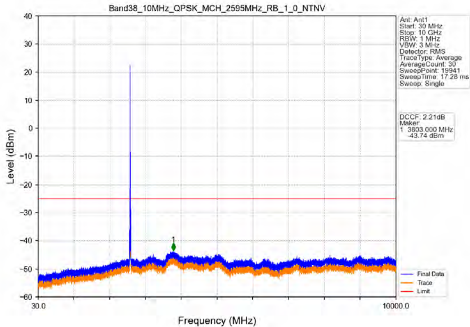
Band38_10MHz_QPSK_MCH_2595MHz_RB_1_0_NTNV
