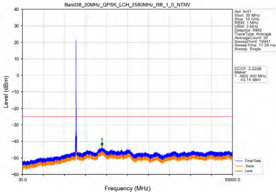
Band38_20MHz_QPSK_LCH_2580MHz_RB_1_0_NTNV
