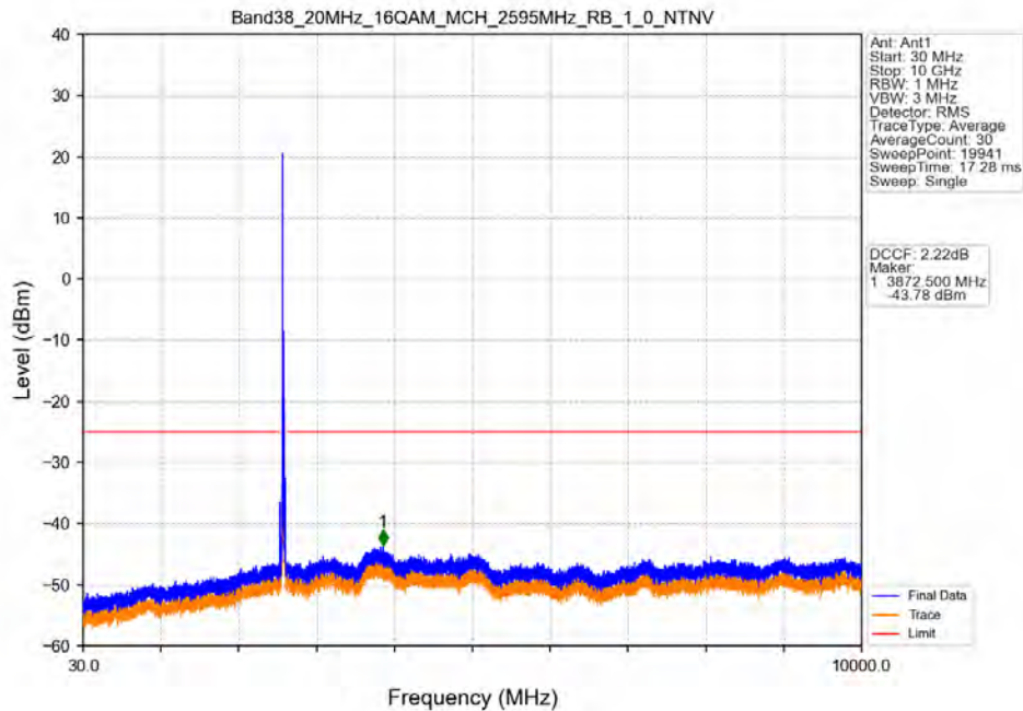
Band38_20MHz_16QAM_MCH_2595MHz_RB_1_0_NTNV
