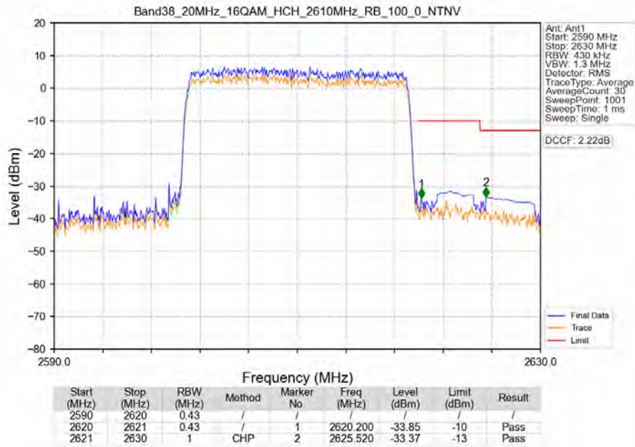
Band38_20MHz_16QAM_HCH_2610MHz_RB_100_0_NTNV
