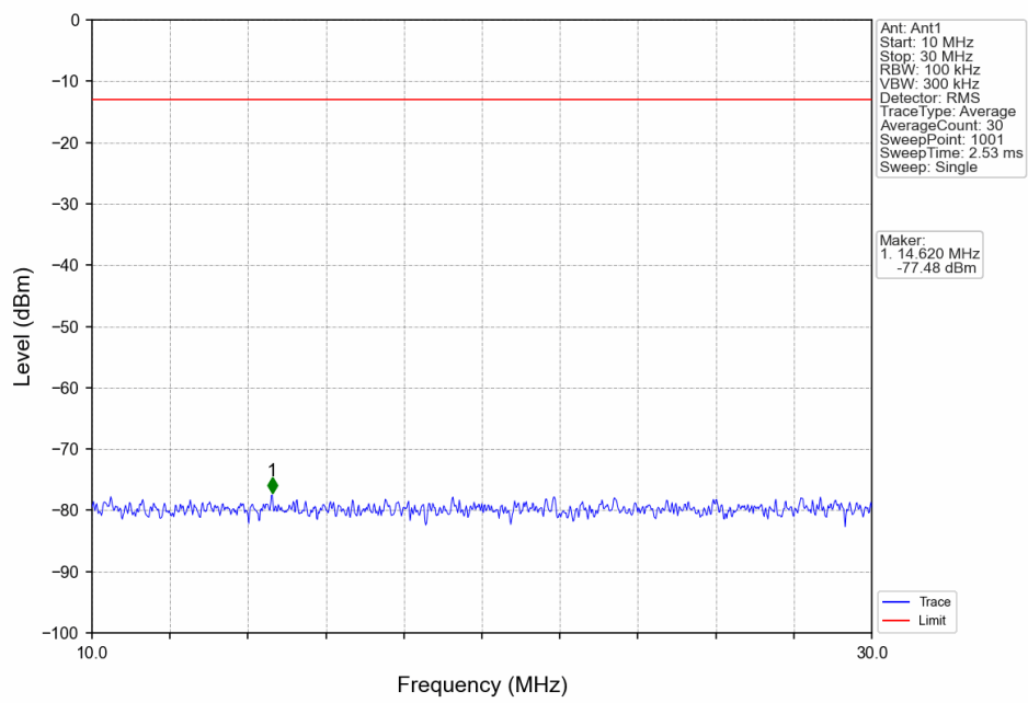
Band71_20MHz_QPSK_HCH_688MHz_RB_1_0_NTNV
