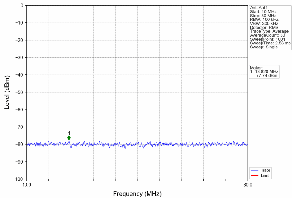
Band71_5MHz_16QAM_LCH_665.5MHz_RB_1_0_NTNV
