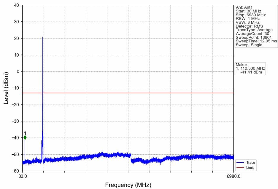
Band71_10MHz_QPSK_HCH_693MHz_RB_1_0_NTNV
