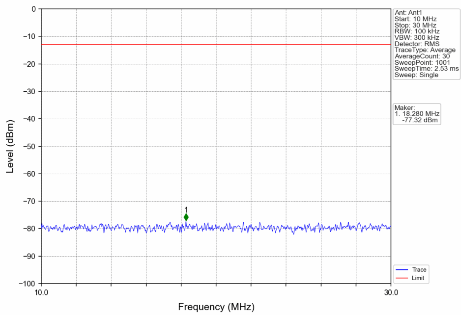
Band71_10MHz_QPSK_HCH_693MHz_RB_1_0_NTNV
