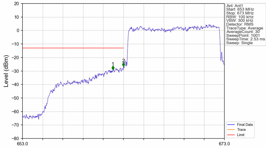
Band71_10MHz_16QAM_LCH_668MHz_RB_50_0_NTNV
