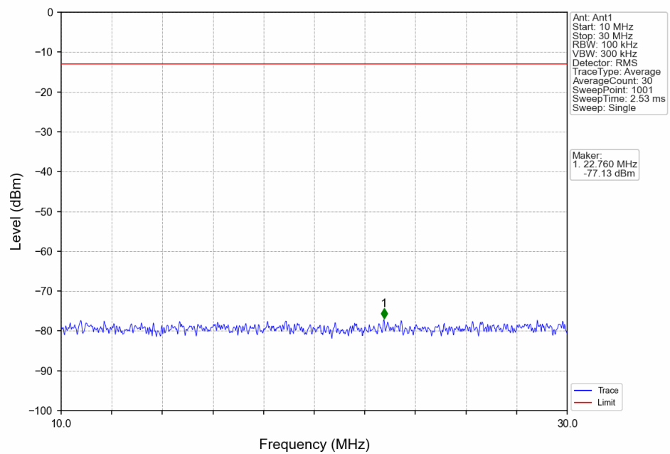
Band71_15MHz_QPSK_LCH_670.5MHz_RB_1_0_NTNV
