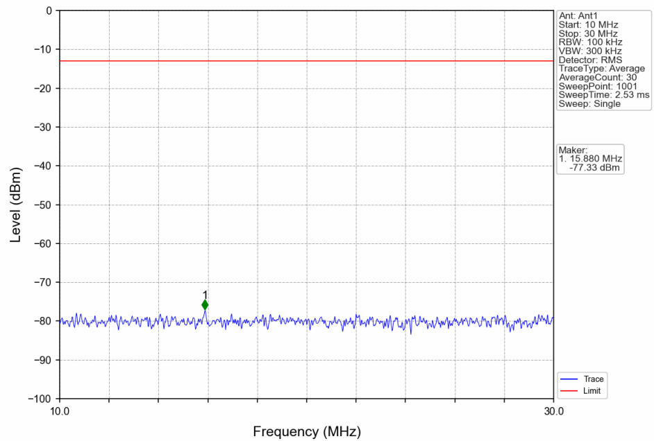
Band71_20MHz_16QAM_LCH_673MHz_RB_1_0_NTNV
