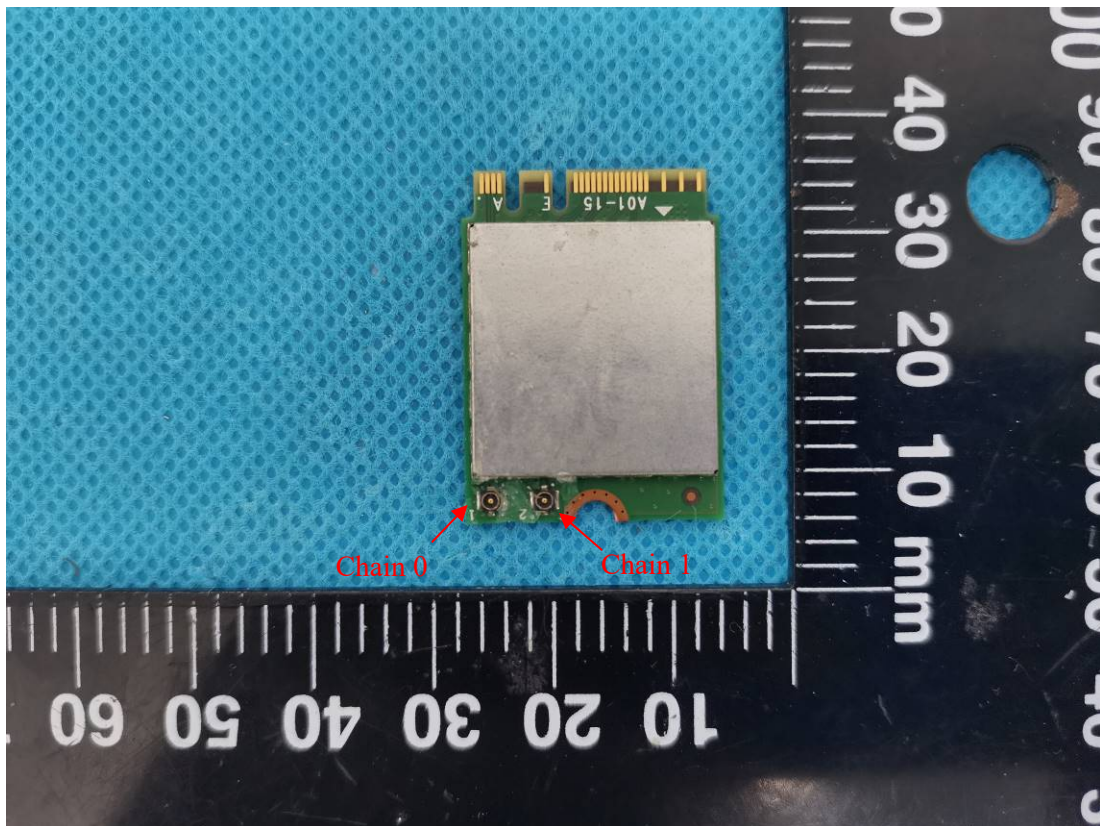
BT/WiFi Module
