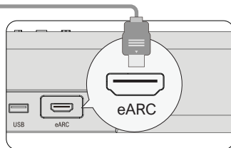
Etape 2: Connectez ensuite l'autre extrémité au port eARC de la barre de son.
