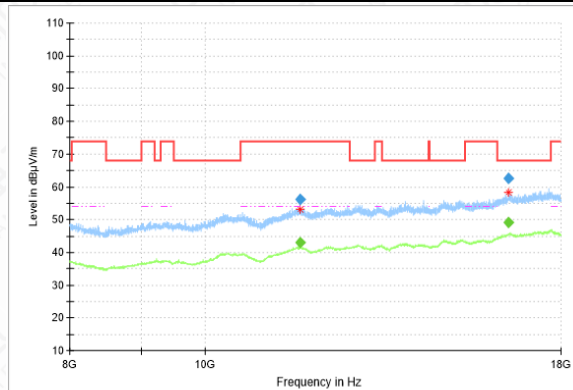
RSE-11AC(80M)-CH155-8GHz-18GHz
