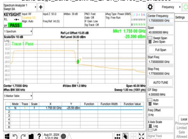
Band Edge_Band4_20MHz_QPSK_RB100_0_CH20300
