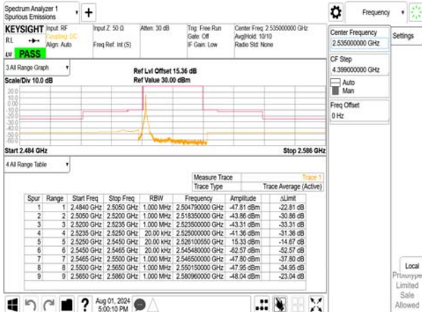
Emission Mask_Band7_20MHz_QPSK_RB1_0_CH21100
