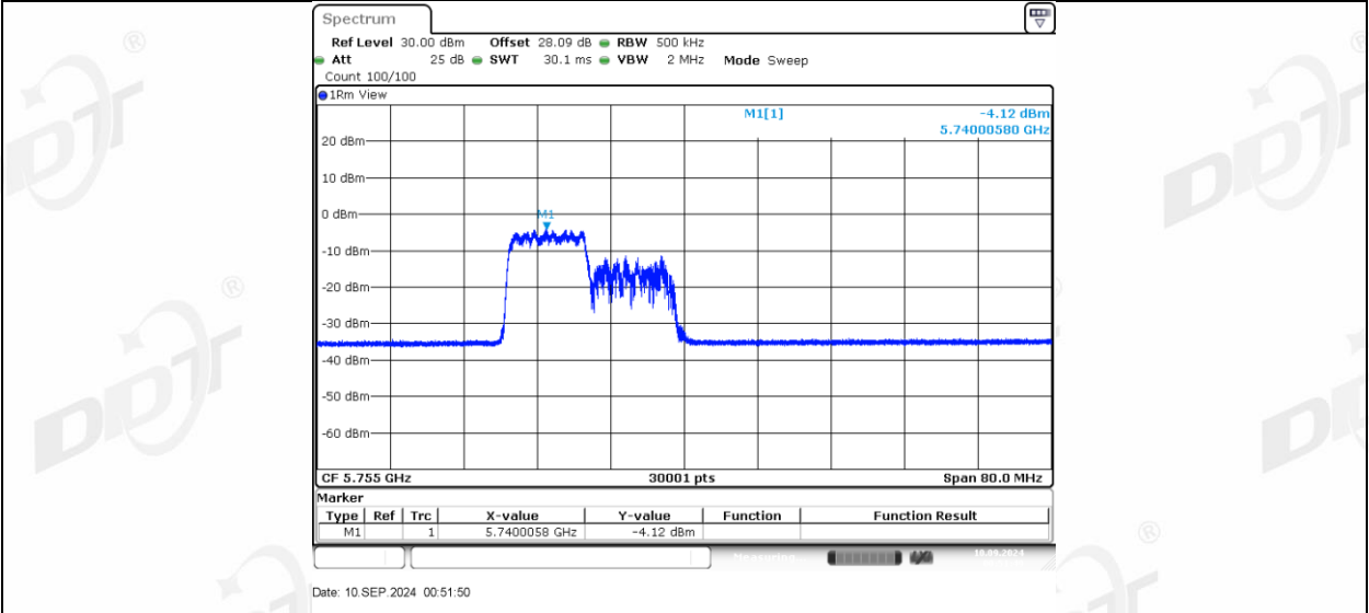
11AX40MIMO_Ant1_5755_106Tone_RU56
