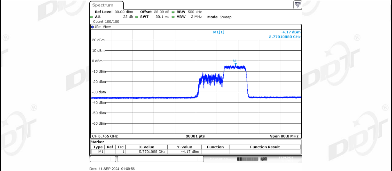
11AX40MIMO_Ant1_5755_242Tone_RU61
