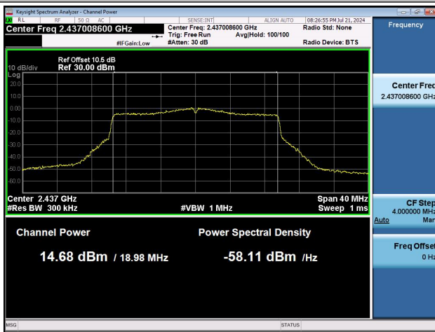
11AX20MIMO-Ant0-2437-PASS
