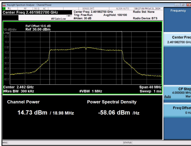
11AX20MIMO-Ant0-2462-PASS
