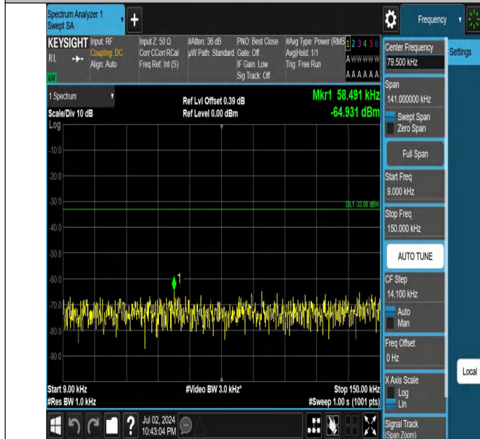
Band5-3MHz-QPSK-20635-1RB#0-0.009~0.15-PASS
