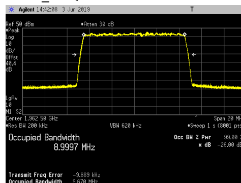
LTE10_16QAM
