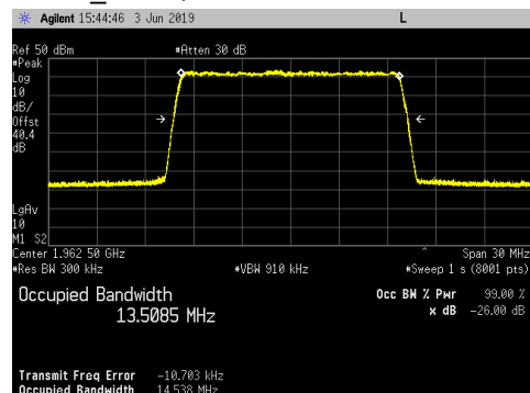
LTE15_256QAM
