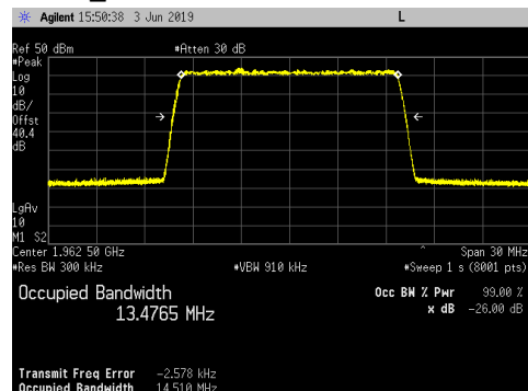
LTE15_QPSK
