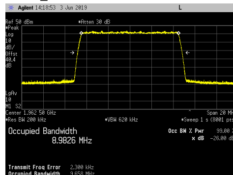
LTE10_QPSK
