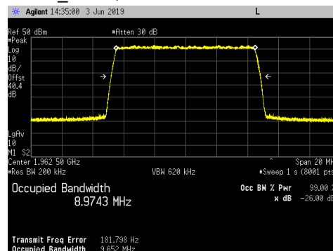
LTE10_256QAM
