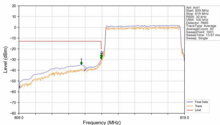
Band26a 5MHz 16QAM LCH 816.5MHz RB 25 0 NTNV
