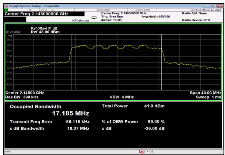
Figure 566: 16QAM 20MHz B.W.; 2145.0MHz, 60kHz - Output
