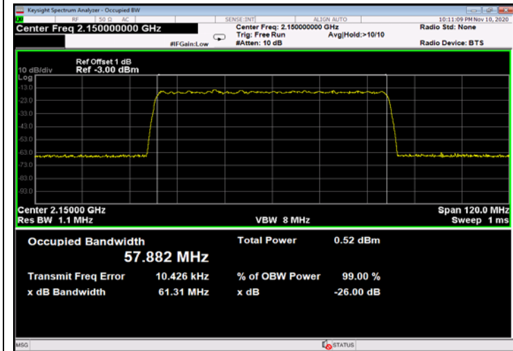
Figure 535: QPSK 60MHz B.W.; 2150.0MHz, 30kHz - Input
