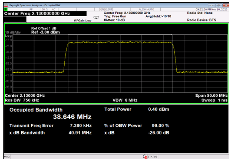
Figure 513: QPSK 40MHz B.W.; 2130.0MHz, 15kHz - Input
