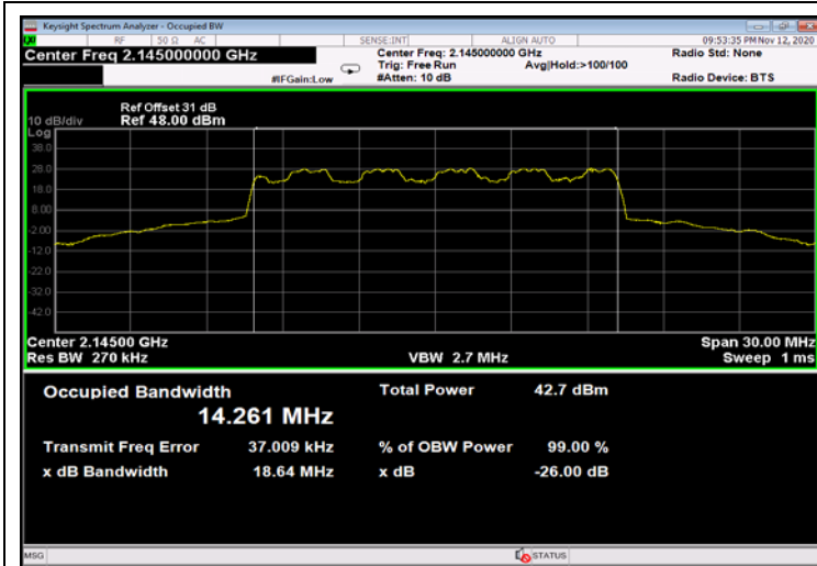
Figure 555: 16QAM 15MHz B.W.; 2145.0MHz, 15kHz - Output
