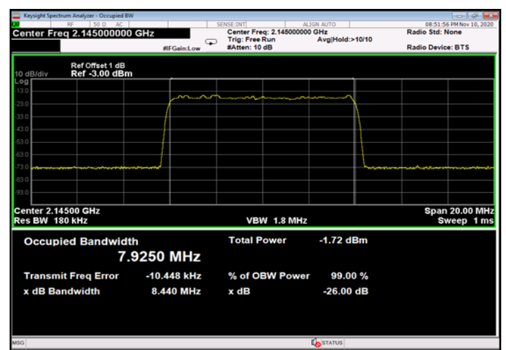
Figure 482: QPSK 10MHz B.W.; 2145.0MHz, 60kHz - Input
