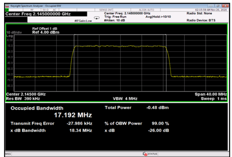
Figure 500: QPSK 20MHz B.W.; 2145.0MHz, 60kHz - Input
