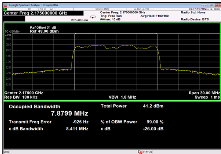
Figure 551: 16QAM 10MHz B.W.; 2175.0MHz, 60kHz - Output
