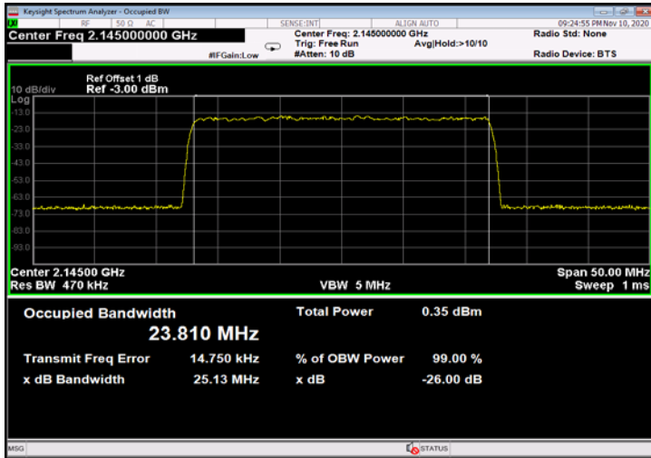
Figure 507: QPSK 25MHz B.W.; 2145.0MHz, 15kHz - Input
