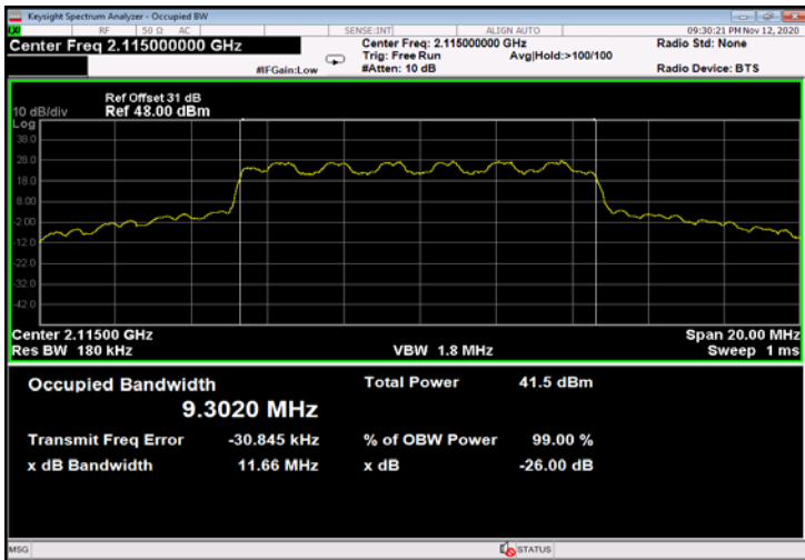
Figure 543: 16QAM 10MHz B.W.; 2115.0MHz, 15kHz - Output
