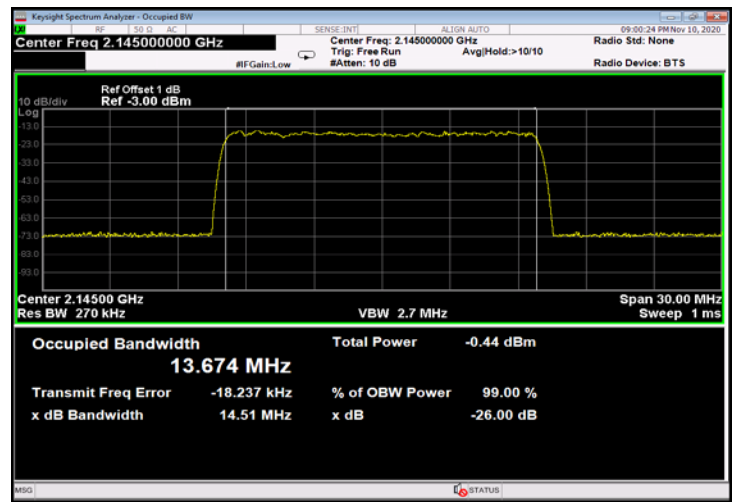
Figure 490: QPSK 15MHz B.W.; 2145.0MHz, 30kHz - Input
