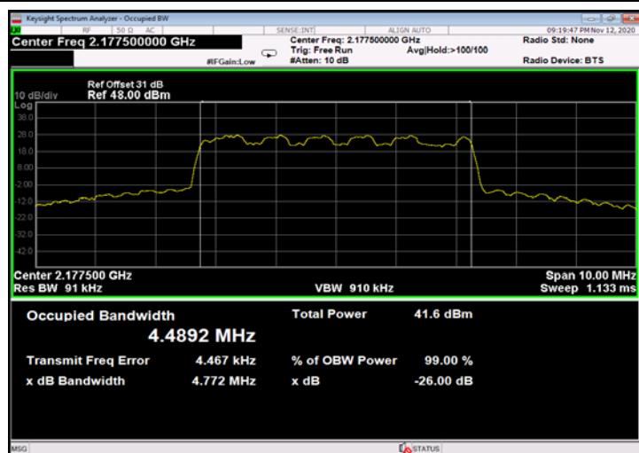
Figure 541: 16QAM 5MHz B.W.; 2177.5MHz, 15kHz - Output
