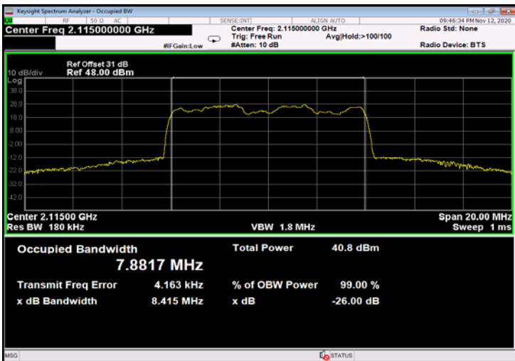
Figure 545: 16QAM 10MHz B.W.; 2115.0MHz, 60kHz - Output
