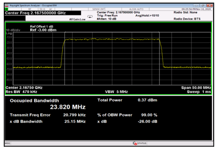
Figure 510: QPSK 25MHz B.W.; 2167.5MHz, 15kHz - Input
