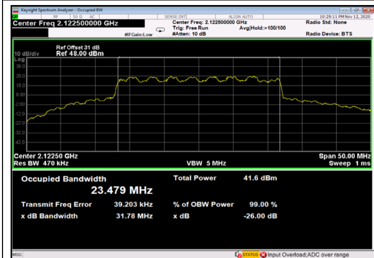
Figure 571: 16QAM 25MHz B.W.; 2122.5MHz, 30kHz - Output
