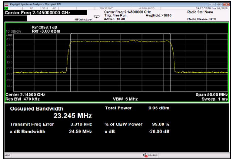
Figure 508: QPSK 25MHz B.W.; 2145.0MHz, 30kHz - Input
