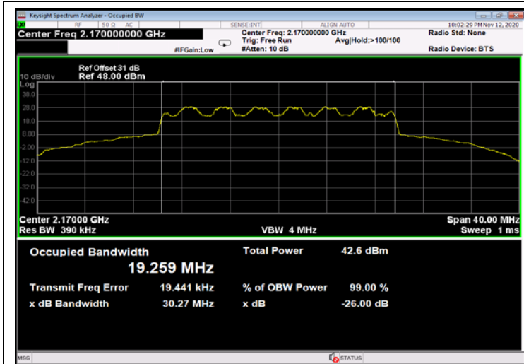
Figure 567: 16QAM 20MHz B.W.; 2170.0MHz, 15kHz - Output
