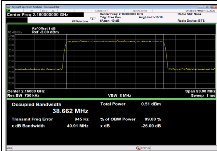
Figure 519: QPSK 40MHz B.W.; 2160.0MHz, 15kHz - Input
