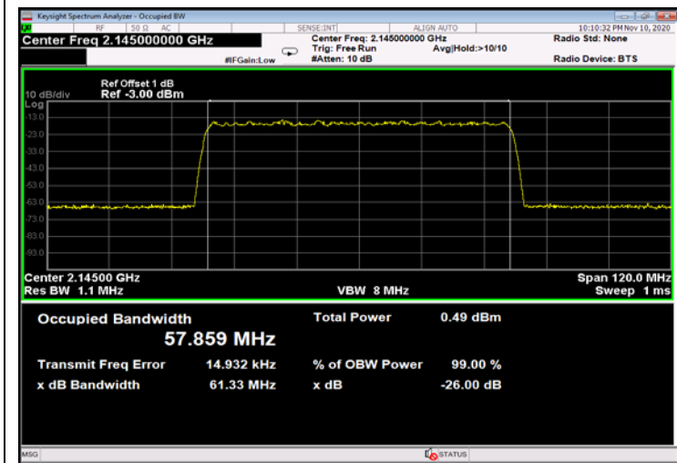
Figure 533: QPSK 60MHz B.W.; 2145.0MHz, 30kHz - Input
