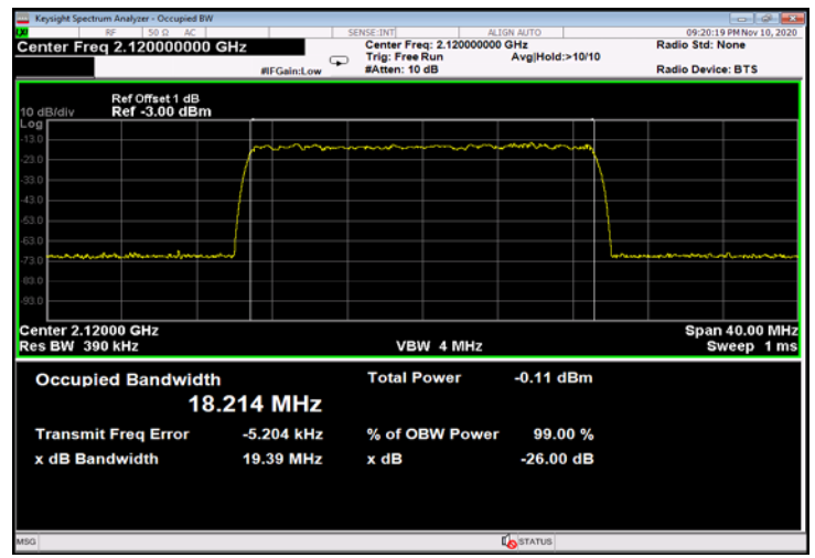
Figure 496: QPSK 20MHz B.W.; 2120.0MHz, 30kHz - Input
