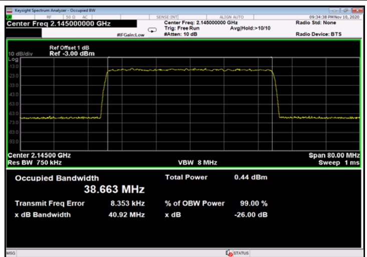
Figure 516: QPSK 40MHz B.W.; 2145.0MHz, 15kHz - Input
