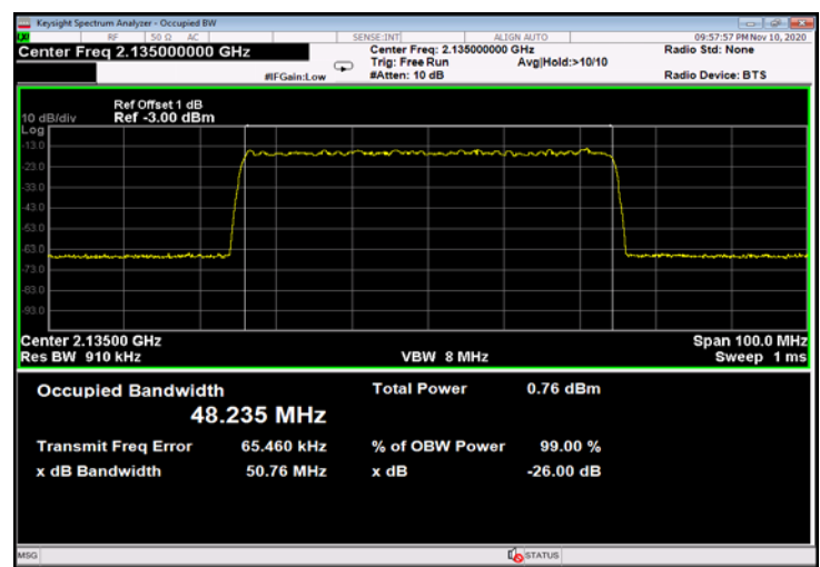
Figure 522: QPSK 50MHz B.W.; 2135.0MHz, 15kHz - Input
