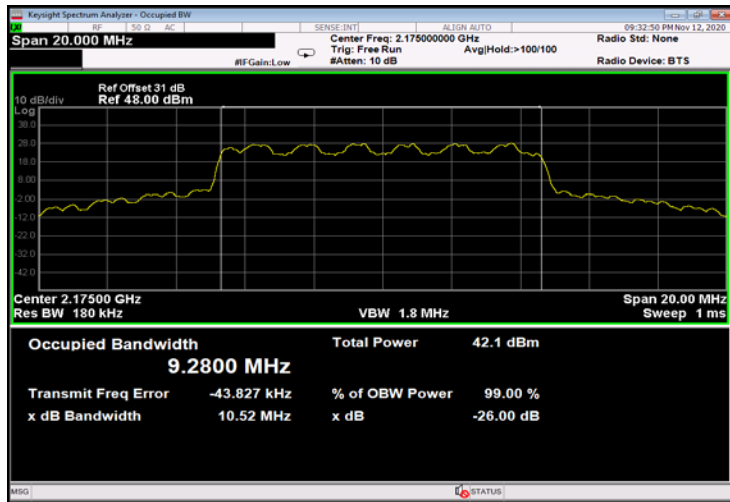
Figure 549: 16QAM 10MHz B.W.; 2175.0MHz, 15kHz - Output
