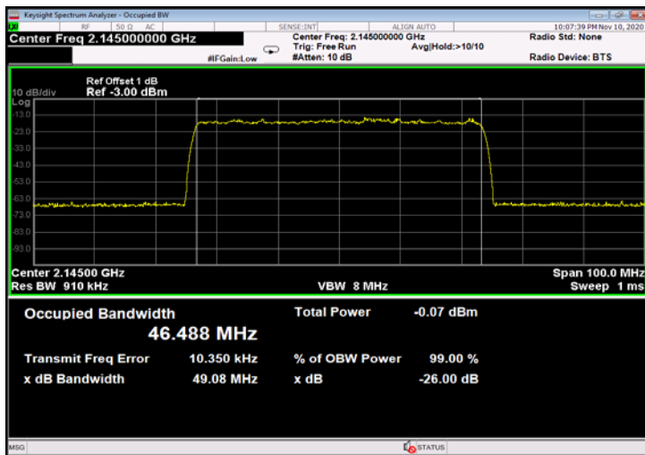
Figure 527: QPSK 50MHz B.W.; 2145.0MHz, 60kHz - Input
