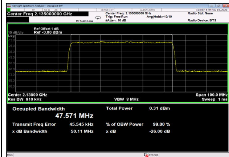
Figure 523: QPSK 50MHz B.W.; 2135.0MHz, 30kHz - Input
