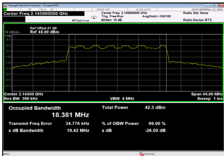
Figure 565: 16QAM 20MHz B.W.; 2145.0MHz, 30kHz - Output
