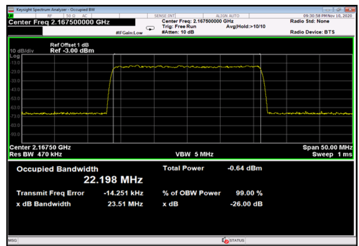
Figure 512: QPSK 25MHz B.W.; 2167.5MHz, 60kHz - Input
