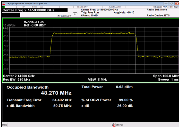
Figure 525: QPSK 50MHz B.W.; 2145.0MHz, 15kHz - Input
