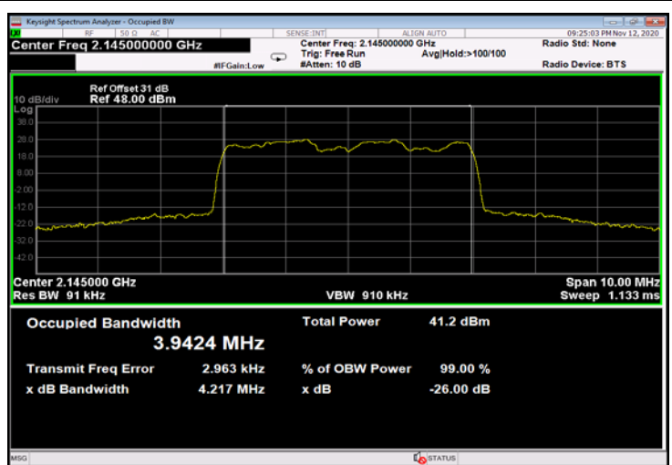
Figure 540: 16QAM 5MHz B.W.; 2145.0MHz, 30kHz - Output
