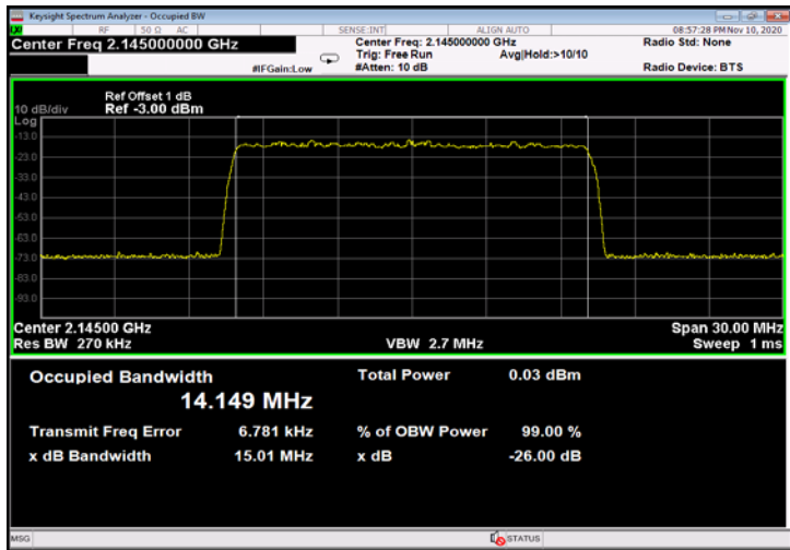
Figure 489: QPSK 15MHz B.W.; 2145.0MHz, 15kHz - Input
