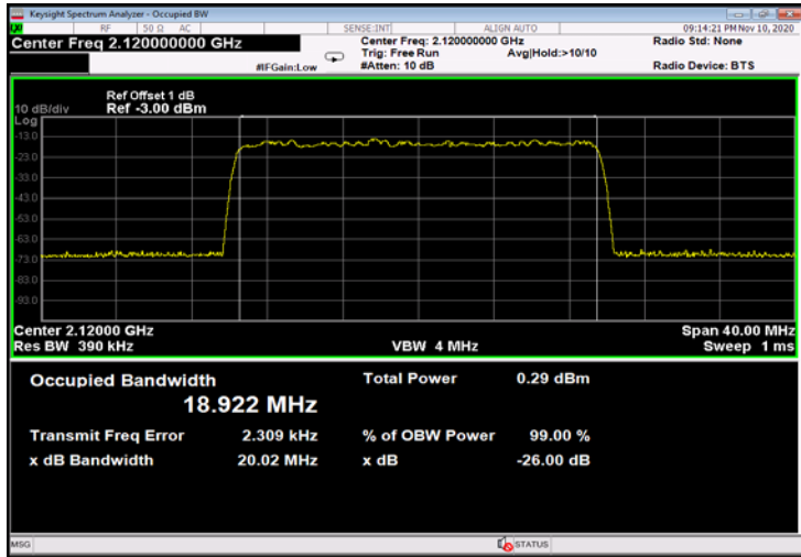
Figure 495: QPSK 20MHz B.W.; 2120.0MHz, 15kHz - Input
