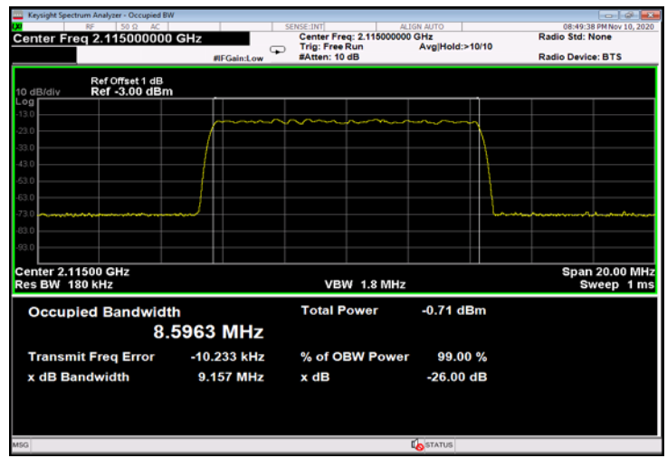
Figure 478: QPSK 10MHz B.W.; 2115.0MHz, 30kHz - Input
