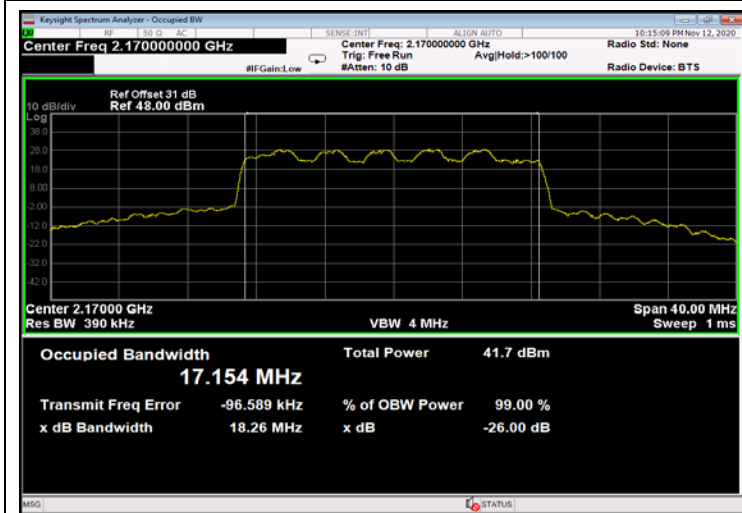
Figure 569: 16QAM 20MHz B.W.; 2170.0MHz, 60kHz - Output
