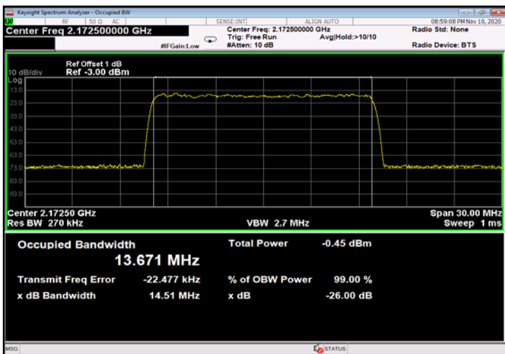
Figure 493: QPSK 15MHz B.W.; 2172.5MHz, 30kHz - Input
