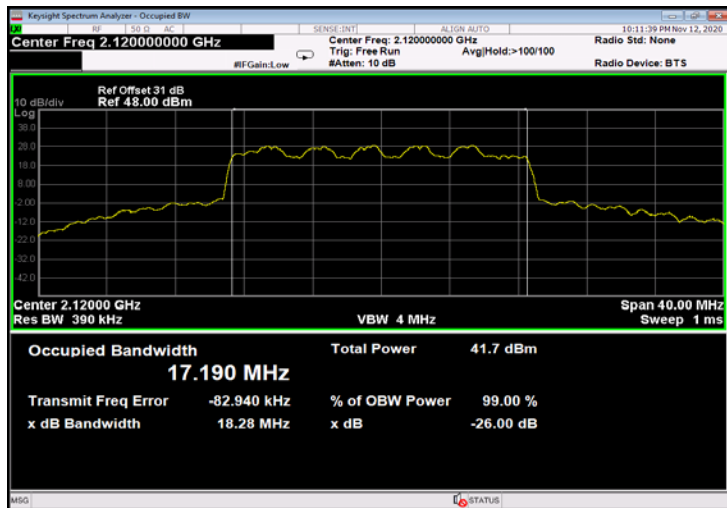
Figure 563: 16QAM 20MHz B.W.; 2120.0MHz, 60kHz - Output
