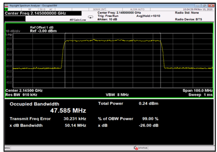
Figure 526: QPSK 50MHz B.W.; 2145.0MHz, 30kHz - Input
