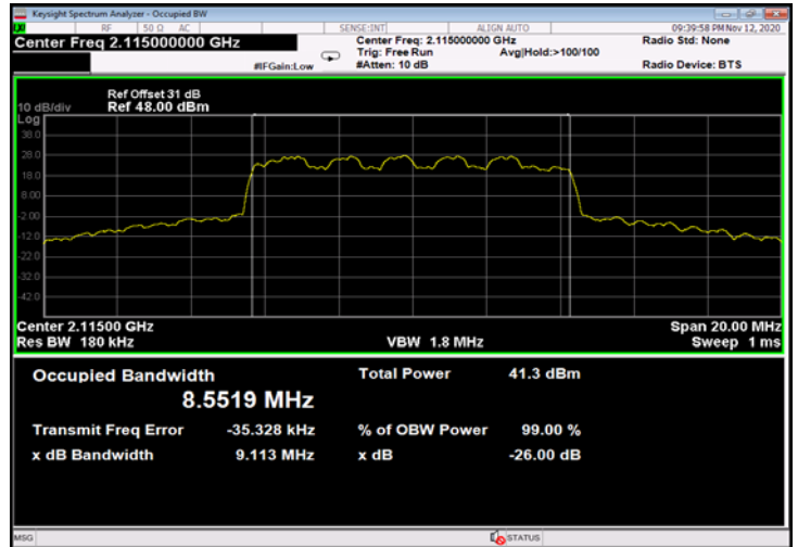
Figure 544: 16QAM 10MHz B.W.; 2115.0MHz, 30kHz - Output
