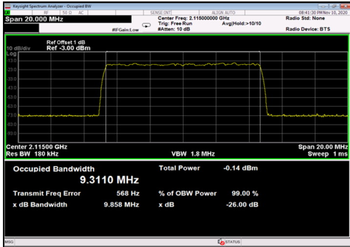
Figure 477: QPSK 10MHz B.W.; 2115.00MHz, 15kHz - Input
