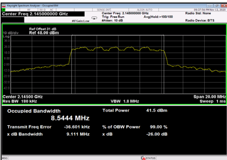
Figure 547: 16QAM 10MHz B.W.; 2145.0MHz, 30kHz - Output
