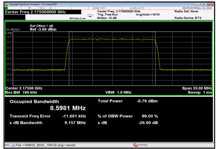
Figure 484: QPSK 10MHz B.W.; 2175.0MHz, 30kHz - Input
