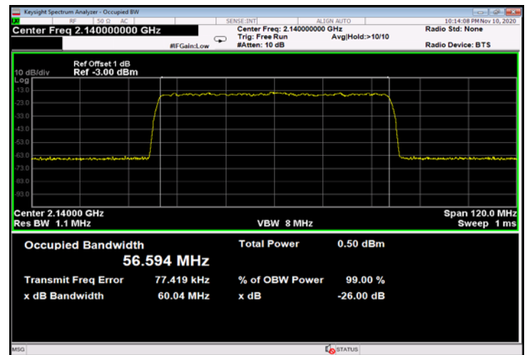
Figure 532: QPSK 60MHz B.W.; 2140.0MHz, 60kHz - Input
