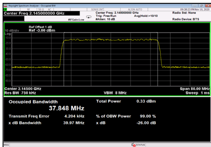
Figure 517: QPSK 40MHz B.W.; 2145.0MHz, 30kHz - Input
