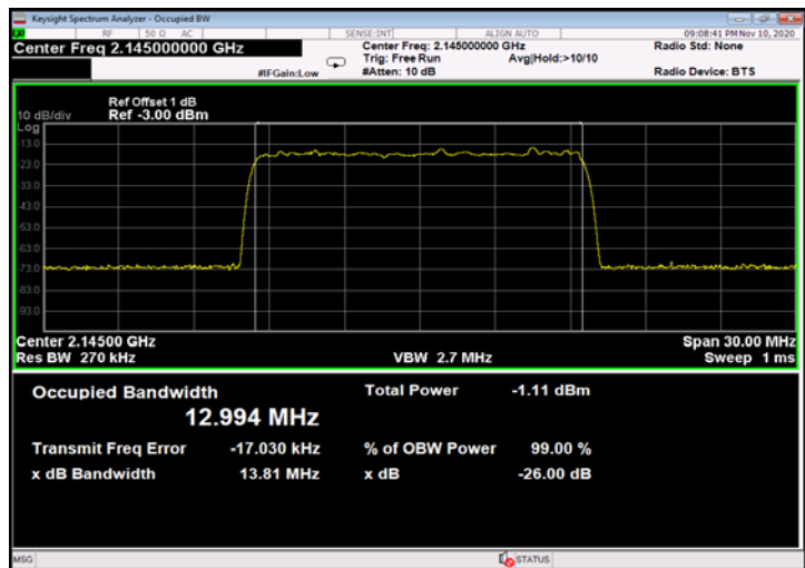
Figure 491: QPSK 15MHz B.W.; 2145MHz, 60kHz - Input
