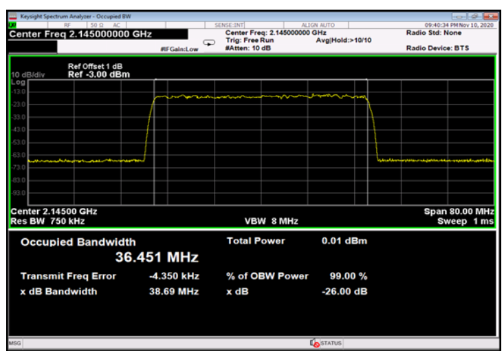
Figure 518: QPSK 40MHz B.W.; 2145.0MHz, 60kHz - Input
