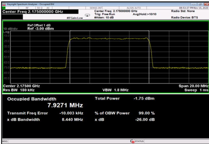
Figure 485: QPSK 10MHz B.W.; 2175.0MHz, 60kHz - Input
