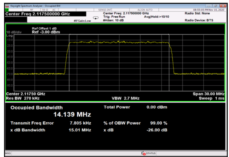
Figure 486: QPSK 15MHz B.W.; 2117.5MHz, 15kHz - Input
