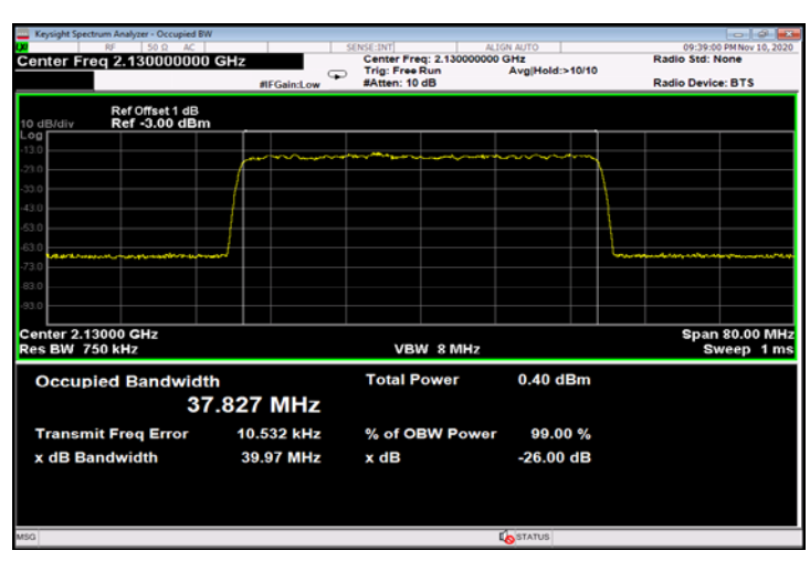
Figure 514: QPSK 40MHz B.W.; 2130.0MHz, 30kHz - Input
