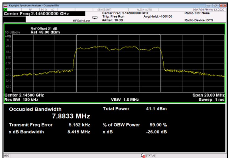
Figure 548: 16QAM 10MHz B.W.; 2145.0MHz, 60kHz - Output
