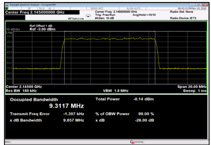
Figure 480: QPSK 10MHz B.W.; 2145.0MHz, 15kHz - Input
