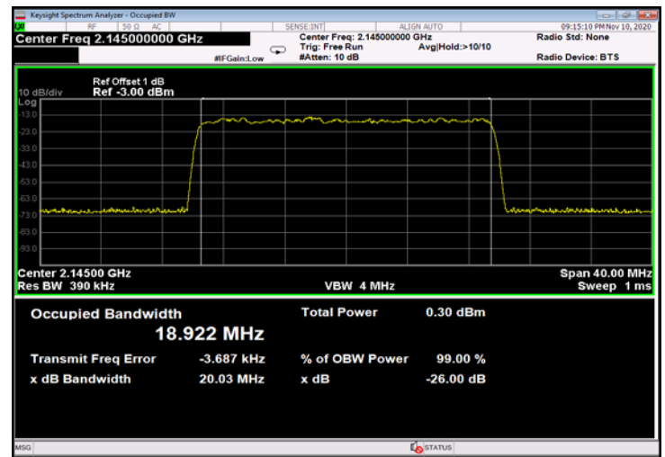
Figure 498: QPSK 20MHz B.W.; 2145.0MHz, 15kHz - Input
