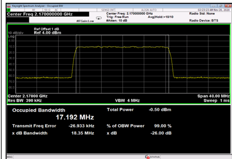
Figure 503: QPSK 20MHz B.W.; 2170.0MHz, 60kHz - Input
