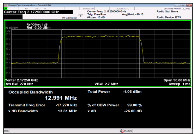
Figure 494: QPSK 15MHz B.W.; 2172.5MHz, 60kHz - Input
