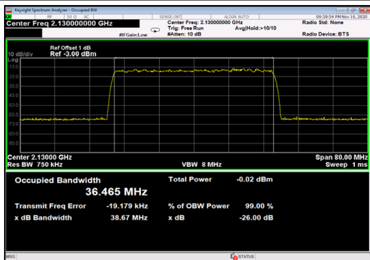
Figure 515: QPSK 40MHz B.W.; 2130.0MHz, 60kHz - Input
