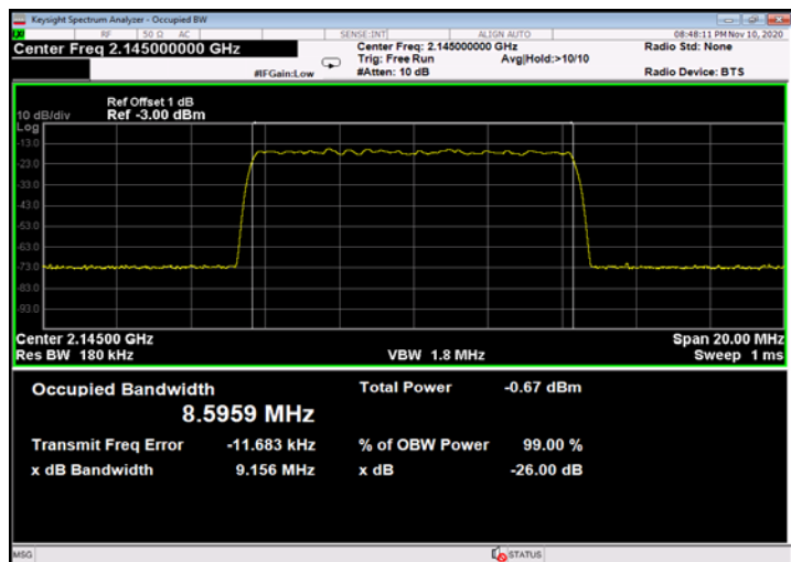
Figure 481: QPSK 10MHz B.W.; 2145.0MHz, 30kHz - Input
