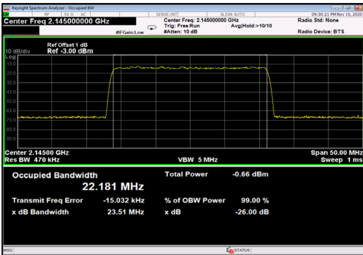
Figure 509: QPSK 25MHz B.W.; 2145.0MHz, 60kHz - Input
