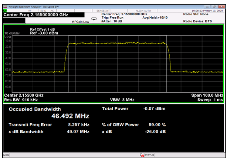
Figure 530: QPSK 50MHz B.W.; 2155.0MHz, 60kHz - Input
