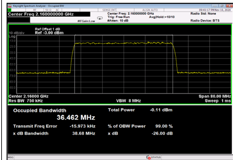
Figure 521: QPSK 40MHz B.W.; 2160.0MHz, 60kHz - Input
