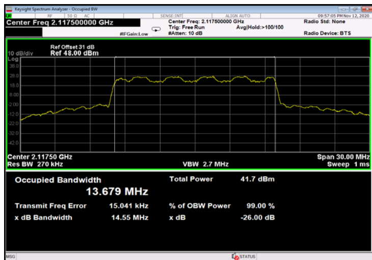
Figure 553: 16QAM 15MHz B.W.; 2117.5MHz, 30kHz - Output
