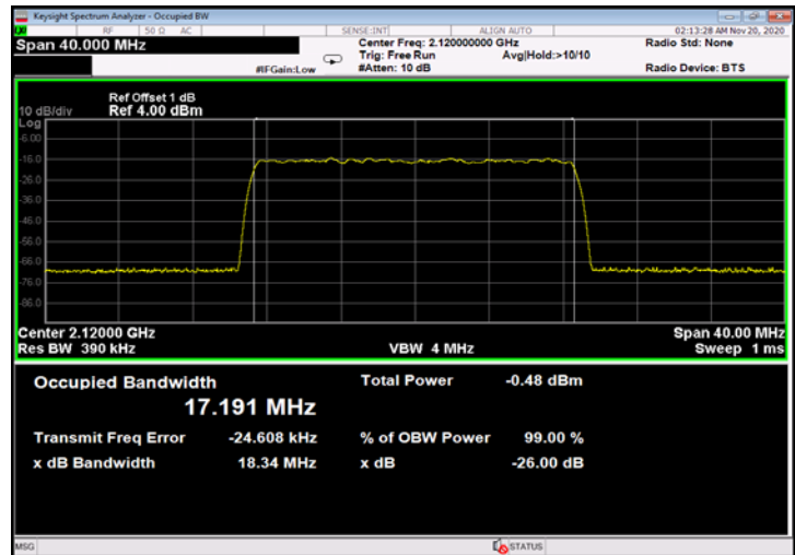
Figure 497: QPSK 20MHz B.W.; 2120.0MHz, 60kHz - Input
