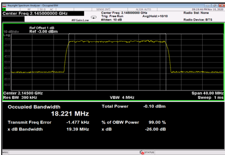
Figure 499: QPSK 20MHz B.W.; 2145.0MHz, 30kHz - Input
