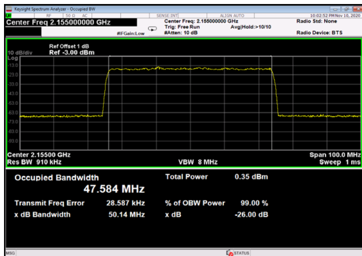
Figure 529: QPSK 50MHz B.W.; 2155.0MHz, 30kHz - Input
