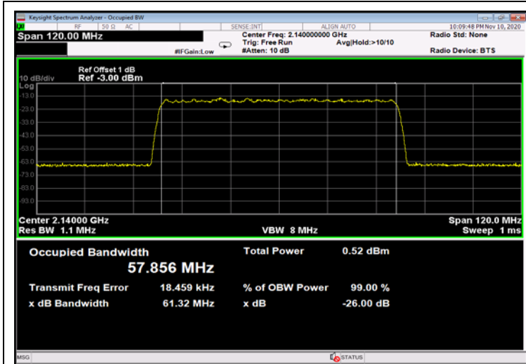
Figure 531: QPSK 60MHz B.W.; 2140.0MHz, 30kHz - Input
