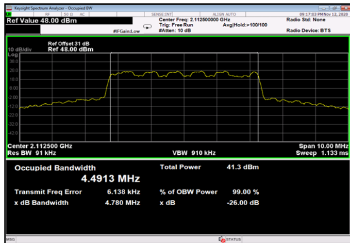
Figure 537: 16QAM 5MHz B.W.; 2112.5MHz, 15kHz - Output
