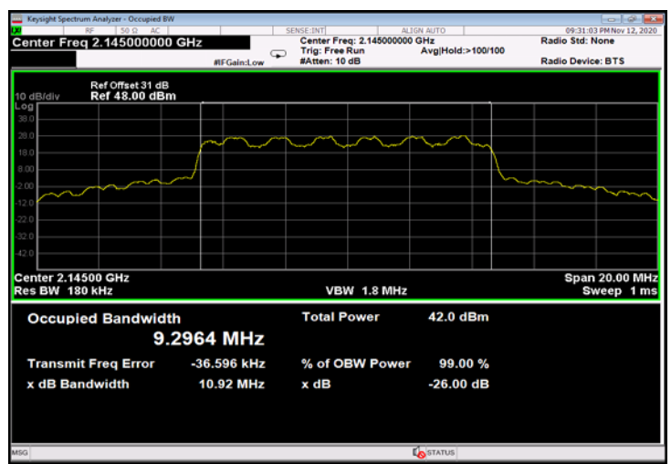
Figure 546: 16QAM 10MHz B.W.; 2145.0MHz, 15kHz - Output
