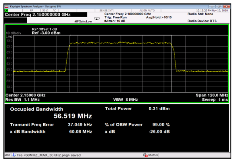
Figure 536: QPSK 60MHz B.W.; 2150.0MHz, 60kHz - Input
