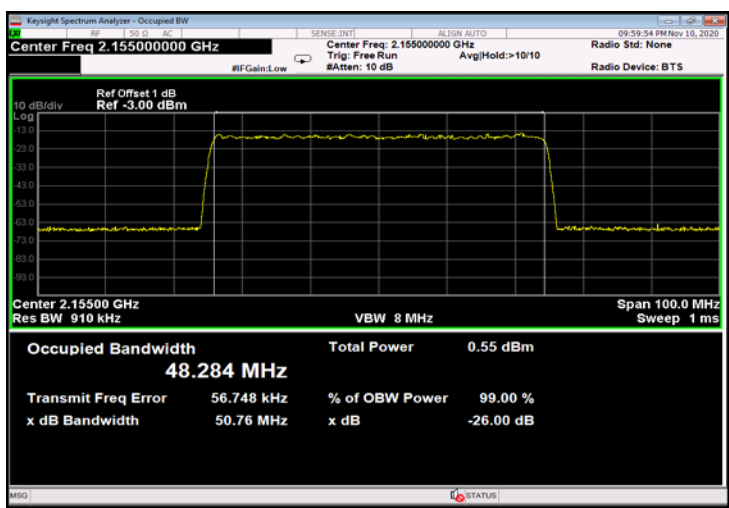
Figure 528: QPSK 50MHz B.W.; 2155.0MHz, 15kHz - Input
