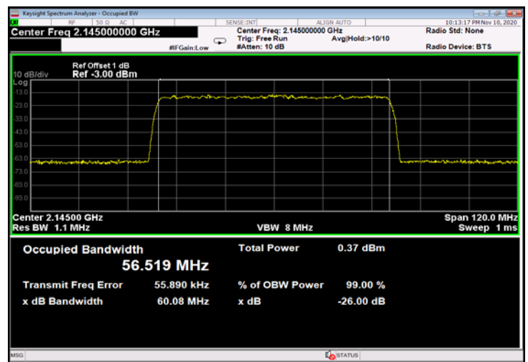
Figure 534: QPSK 60MHz B.W.; 2145.0MHz, 60kHz - Input
