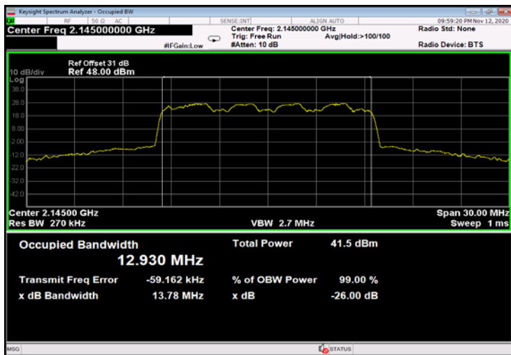
Figure 557: 16QAM 15MHz B.W.; 2145.0MHz, 60kHz - Output
