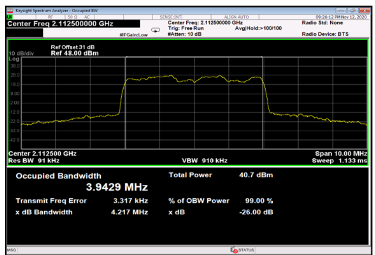
Figure 538: 16QAM 5MHz B.W.; 2112.5MHz, 30kHz - Output
