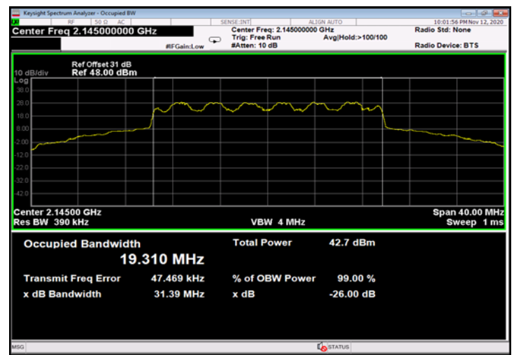
Figure 564: 16QAM 20MHz B.W.; 2145.0MHz, 15kHz - Output
