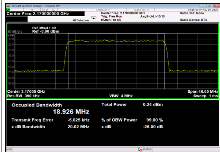
Figure 501: QPSK 20MHz B.W.; 2170.0MHz, 15kHz - Input
