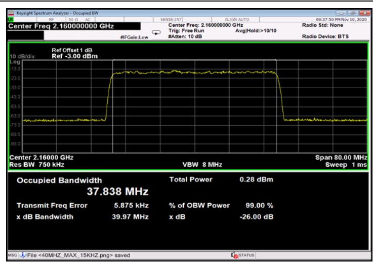
Figure 520: QPSK 40MHz B.W.; 2160.0MHz, 30kHz - Input
