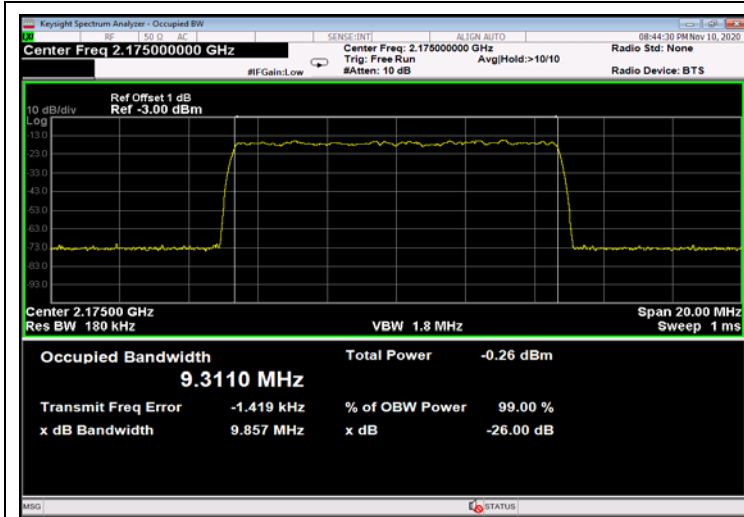
Figure 483: QPSK 10MHz B.W.; 2175.0MHz, 15kHz - Input
