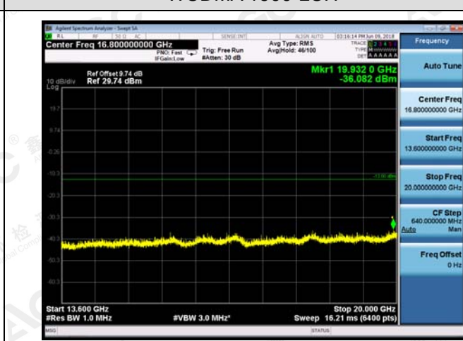
WCDMA 1900-LCH
