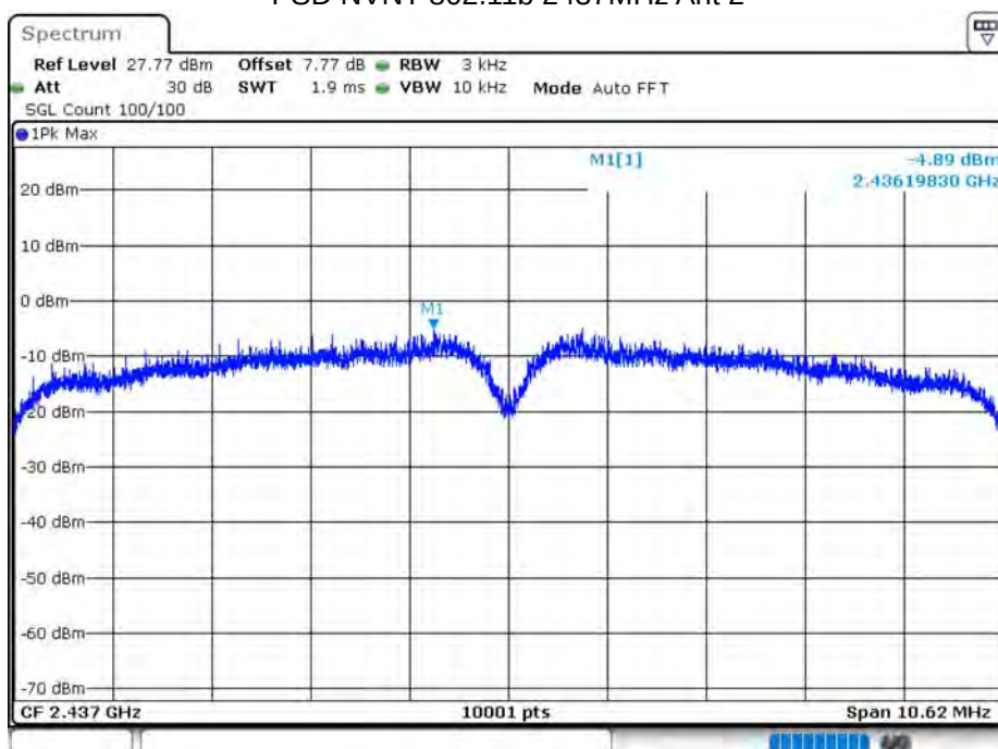
PSD NVNT 802.11b 2437MHz Ant 2
