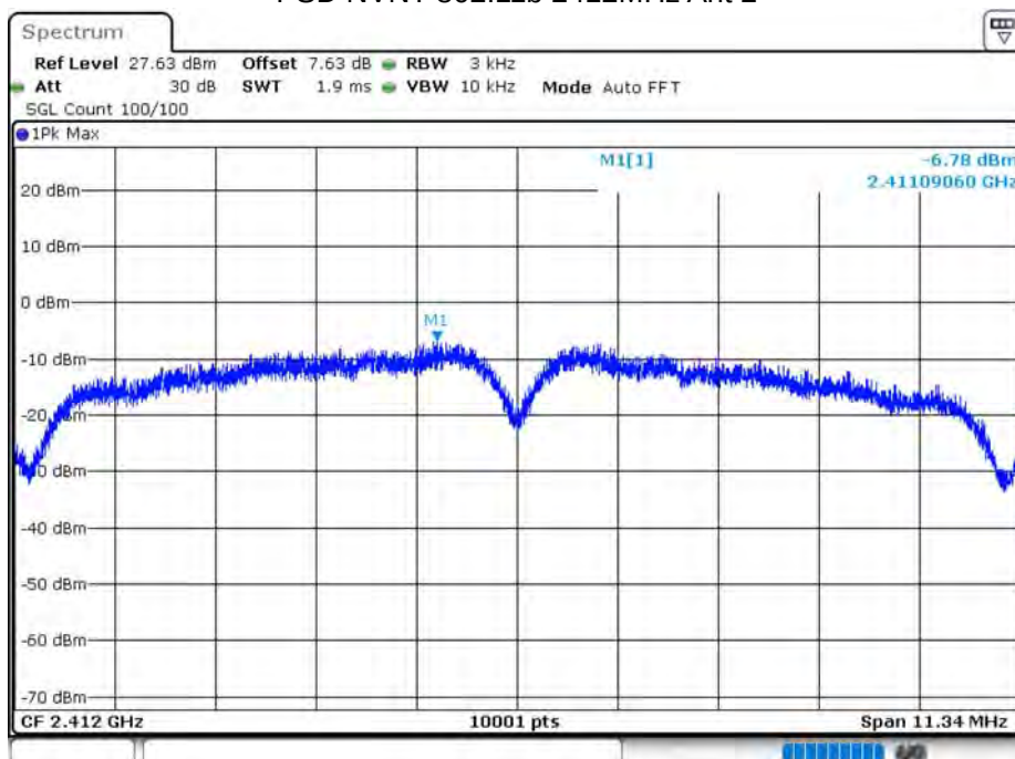
PSD NVNT 802.11b 2412MHz Ant 2
