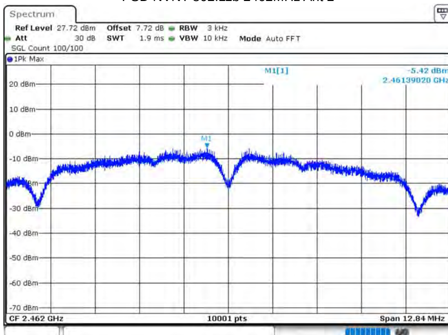
PSD NVNT 802.11b 2462MHz Ant 2
