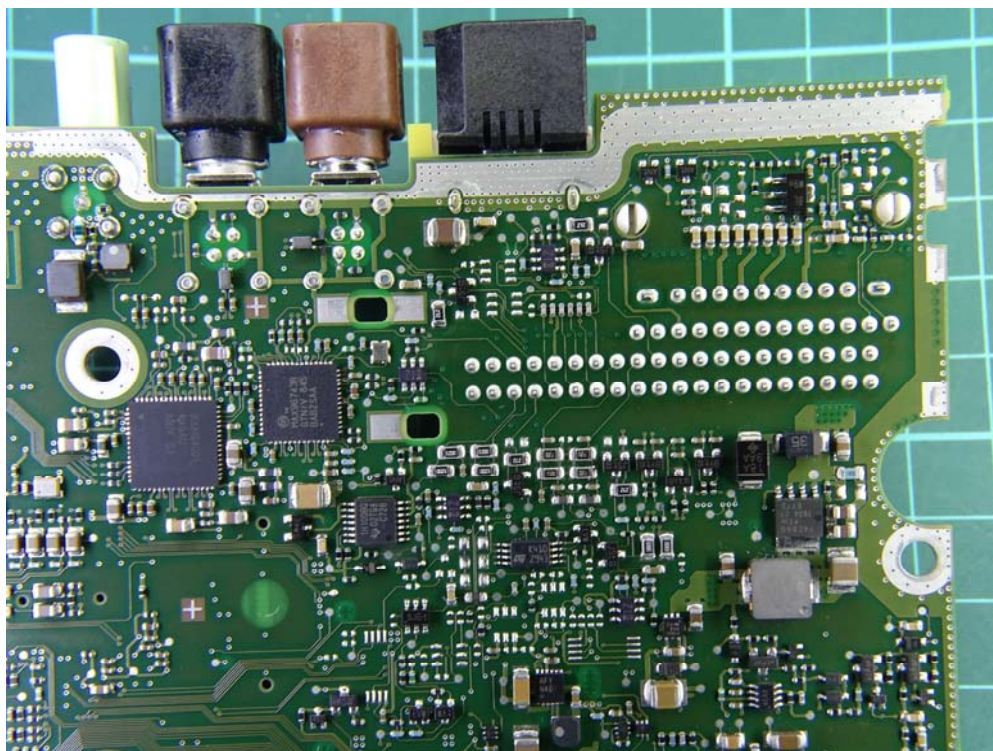
(33) EUT Photo
