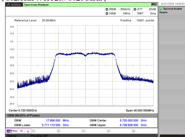
[ 802.11ac (VHT20)/ 5720 MHz ]
