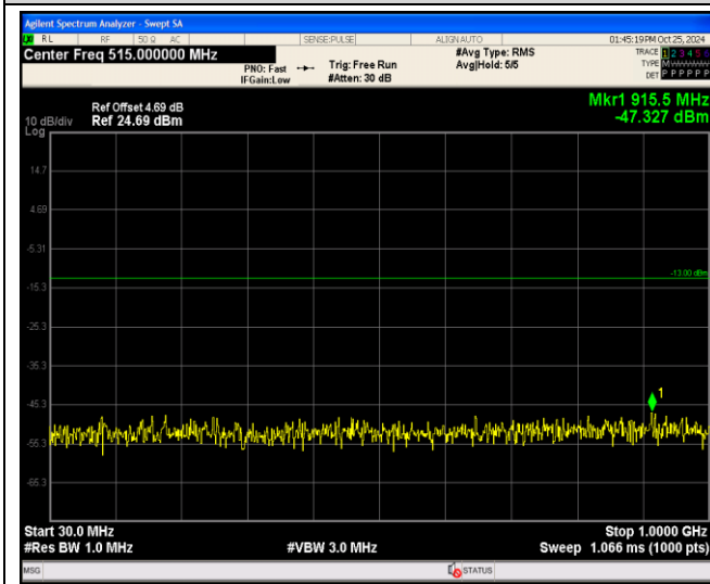
Band2-20MHz-QPSK-18700-1RB#0-Range1:30~1000MHz
