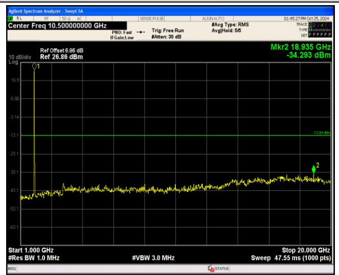
Band2-20MHz-QPSK-18700-1RB#0-Range2:1000~20000MHz
